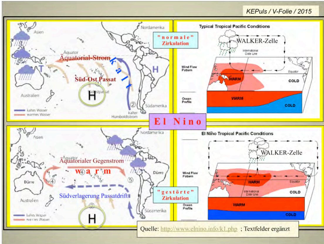
Abb. 2 : LaNina-EINino-Schema
