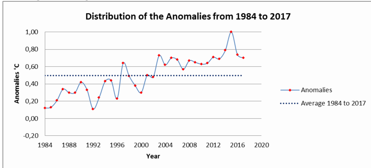
Abbildung 4: Verteilung der Anomalien von 1984 bis 2017
