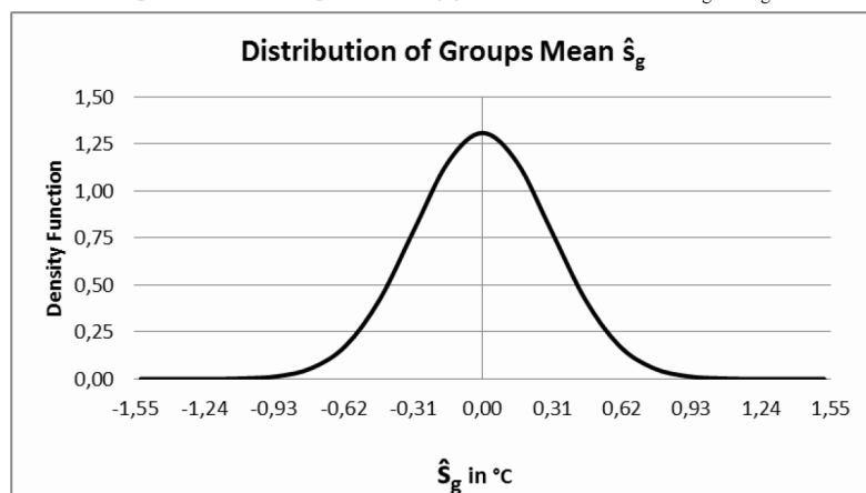
Abbildung 2: Verteilung der Gruppen-Mittelwerte \bar{d}_g = \hat{s}_g
