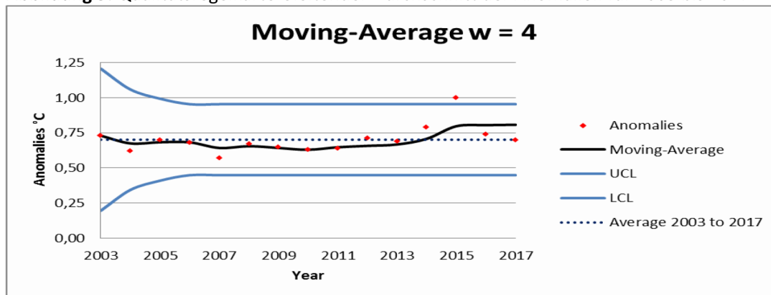
Abbildung 5: Qualitätsregelkarte Gleitender Durchschnitt der Anomalien für 2003 bis 2017
