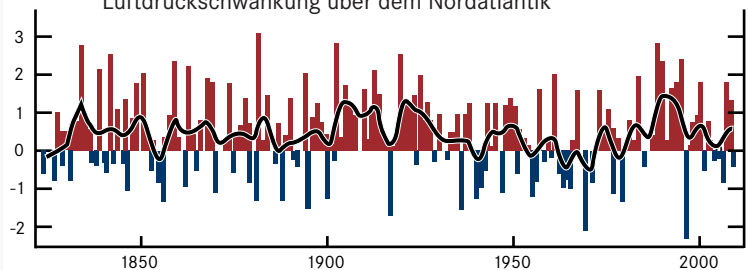
Abb. 1) NAO Index Winter 1820-2009: Luftdruckschwankung über dem Nordatlantik
