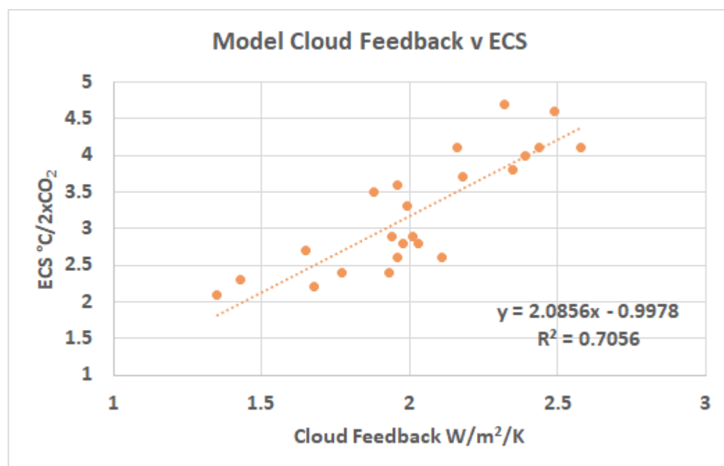
Abbildung 7. Modellierte Wolkenrückkopplung ( \lambda ) aufgetragen gegen modellgeleitetes ECS. Daten aus (Ceppi, Brient, Zelinka, & Hartmann, 2017).
