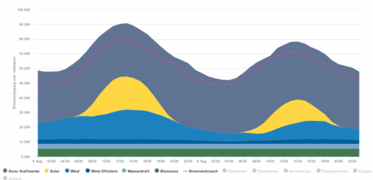
Abb. 8: Sehr viel Sonne und mehr Wind gegen Mittag am 08. und 09.08.2016 („Mittags-Schwemme“). Aber selbst da mussten noch erhebliche Strommengen konventionell erzeugt werden, besonders in den Nächten war deren Anteil sehr hoch. (Bildquelle: Agora Energiewende)
