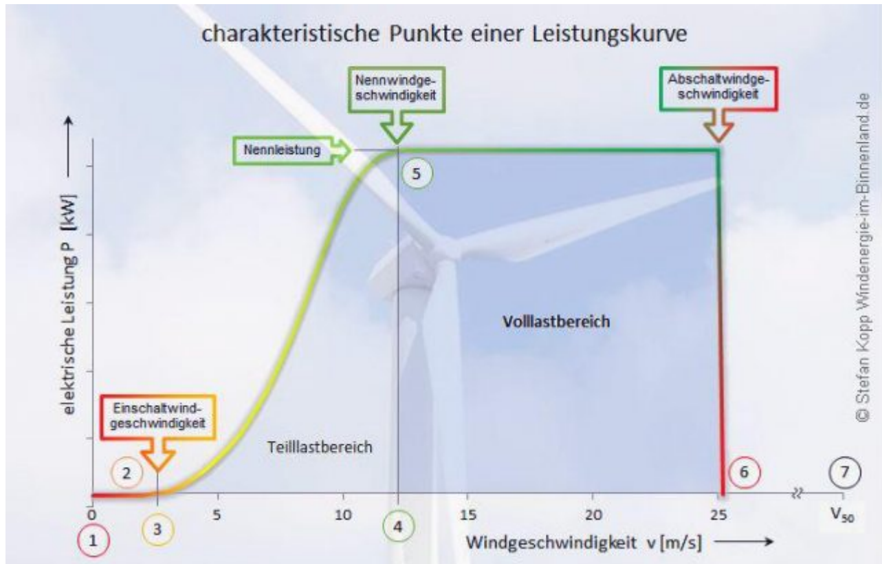
Abb. 2: Unterhalb von 3 m/s, also schwachem Wind, der aber immerhin schon mit ca. 10 Km/h die doppelte Geschwindigkeit eines Fußgängers hat und 1 bis 2 Beaufort entspricht, wird gar kein Strom erzeugt. Danach verachtfacht (!) sich die Leistungsabgabe mit der Verdoppelung der Windgeschwindigkeit („Kubisches Gesetz“), bis erst zwischen 40 und 45 Km/h (etwa 12 bis 13 m/s oder 6 Beaufort) die Nennleistung erreicht wird, welche trotz weiter steigender Windgeschwindigkeit nur noch gleich bleibt. Bei Sturm (25 m/s sind 90 Km/h, das entspricht 10 Beaufort) schalten sich Windräder ab; dieser besonders starke Wind, der gar nicht so selten ist, kann also gar nicht genutzt werden. Bildquelle Stefan Kopp.
