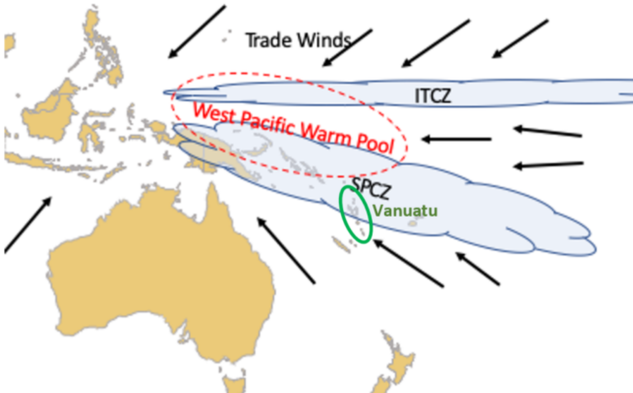
Bild 17 Konvergenzonen im Pazifik. Grafik vom Autor ergänzt. Quelle: South Pacific Convergence Zone (SPCZ) – SKYbrary Aviation Safety
