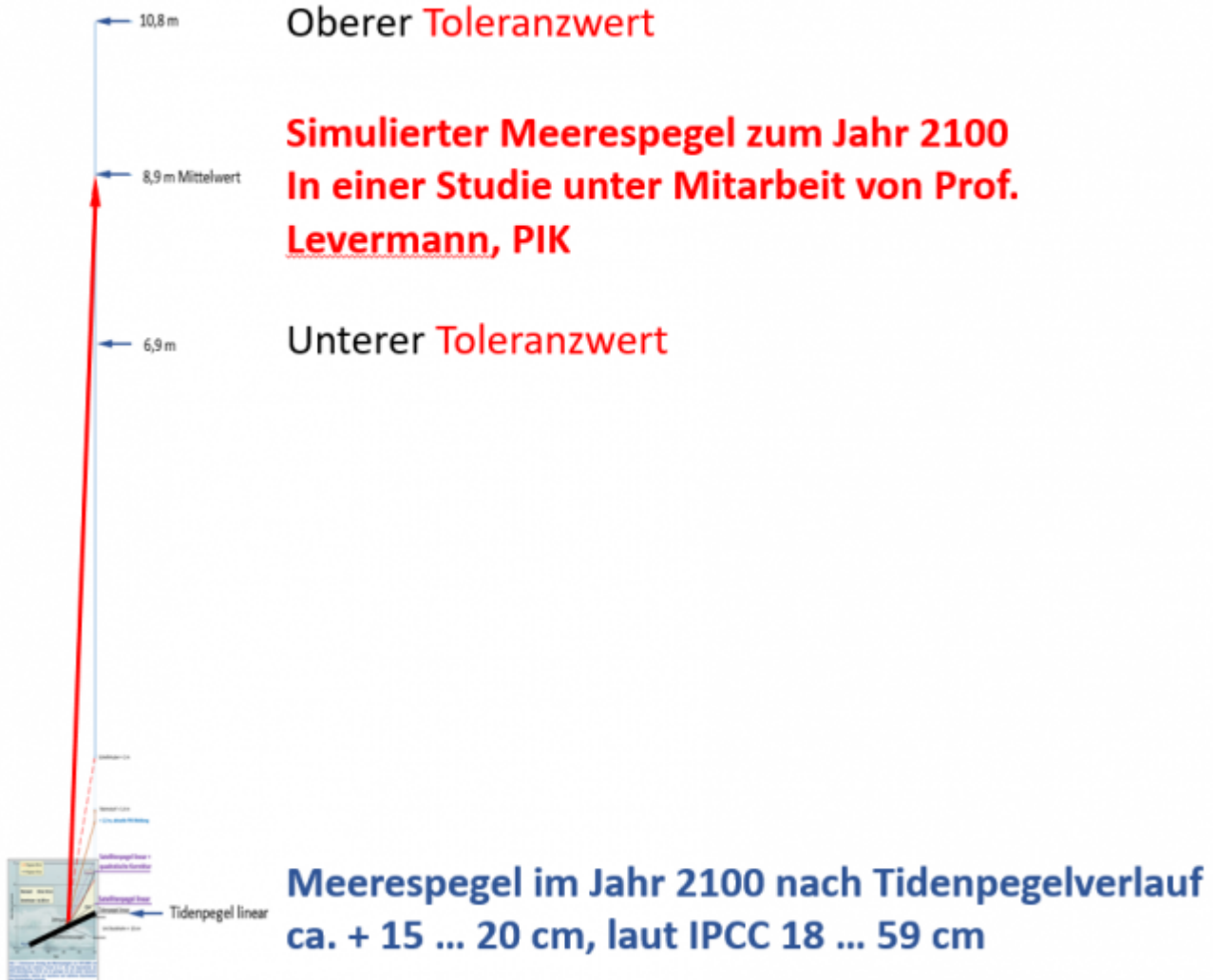
Bild 4 Meeresspiegel-Simulationsvariante aus einer Studie unter Teilnahme des PIK. Beachten: Das kleine, blaue Rechteck ist in etwa maßstabsgetreu die Grafik von Bild 3.
