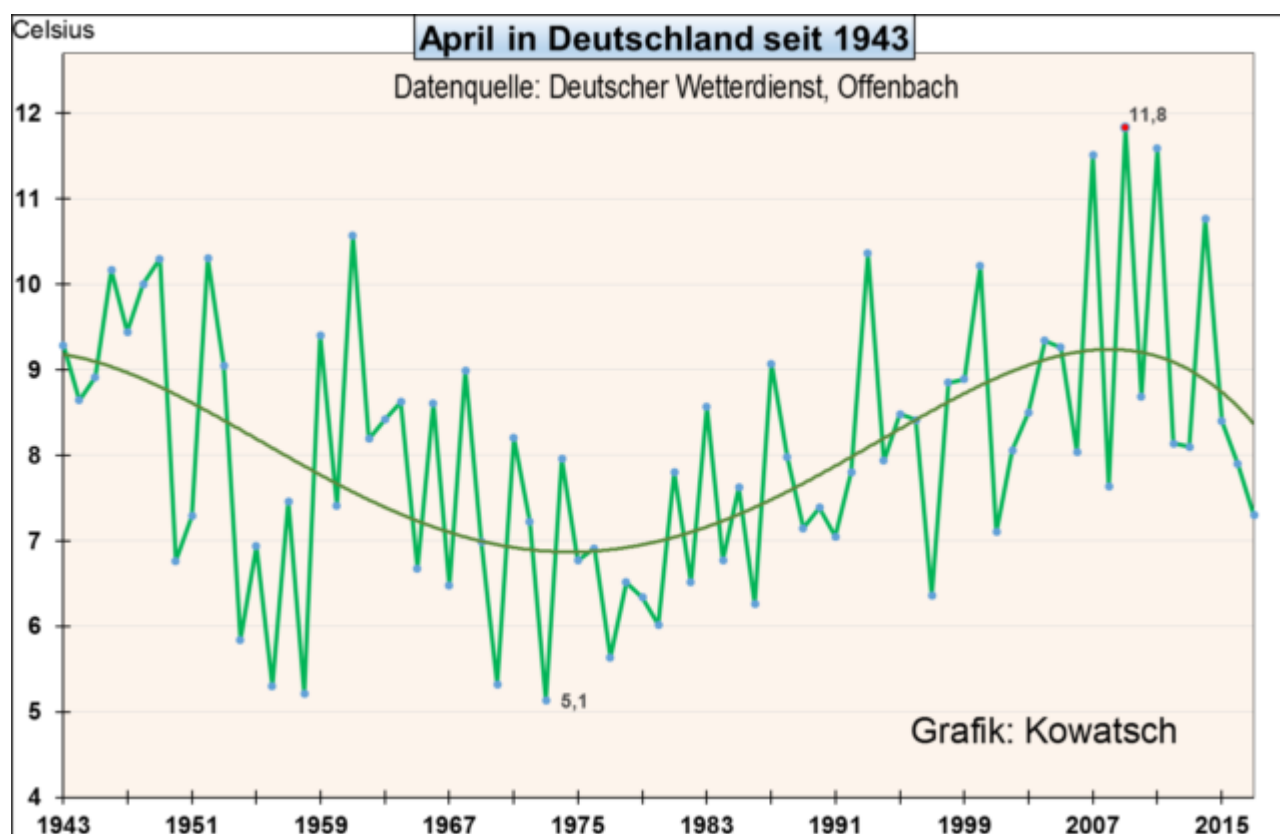
Graphik 3: Auch die Temperaturkurve des Monats April verläuft nicht gleichmäßig, sondern in Form einer Wellenlinie. Während des Krieges hatte der April einen Temperaturwellenberg, der dann in eine allmähliche Abkühlung überging. Nach einer erneuten Erwärmung erreichte der Monat dann 2009 mit 11,8 C einen Temperaturhöhepunkt. Seitdem wird der Monat wieder kälter.
