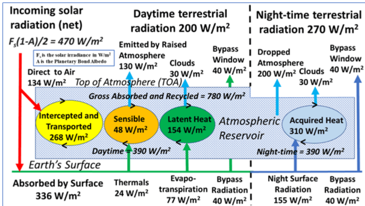
Abbildung 1: Der Prozess der Energieerückgewinnung aus atmosphärischen Reservoiren
