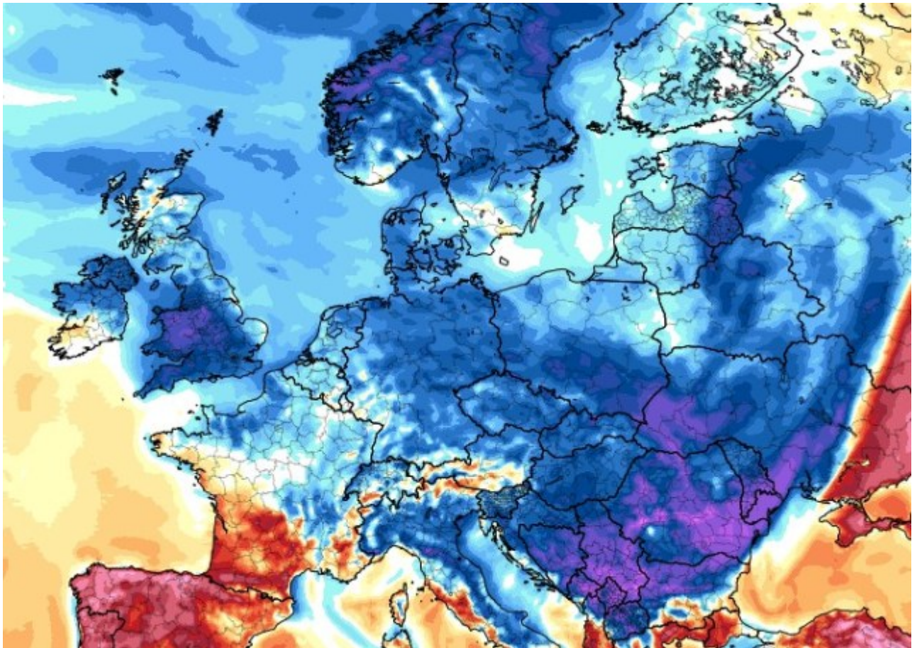
Temperatur-Anomalien in 2 m Höhe vom 11. September (nach GFS; tropicaltidbits.com ).
