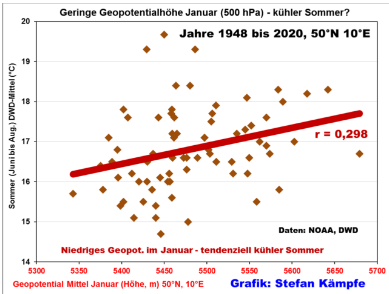
Abbildung 1: Tendenziell kühlere Sommer bei geringerer Höhenlage der 500hPa-Fläche über Deutschland im Januar. Der Zusammenhang ist jedoch für seriöse Vorhersagen viel zu schwach; man achte auf die große Streuung.
