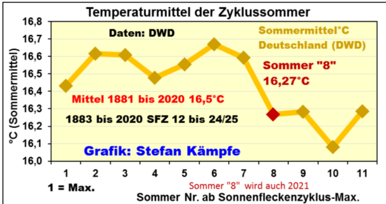
Abbildung 3: Der achte Sommer nach dem Maximum des SCHWABE-Sonnenzyklus verlief im Mittel mit knapp 16,3°C etwas zu kalt; unter diesen befinden sich solche sehr kühlen wie 1913, 1954, 1965 und 1987; mit 1976, 1997 und 2009 aber auch zumindest phasenweise warme, extrem warme fehlen jedoch.
