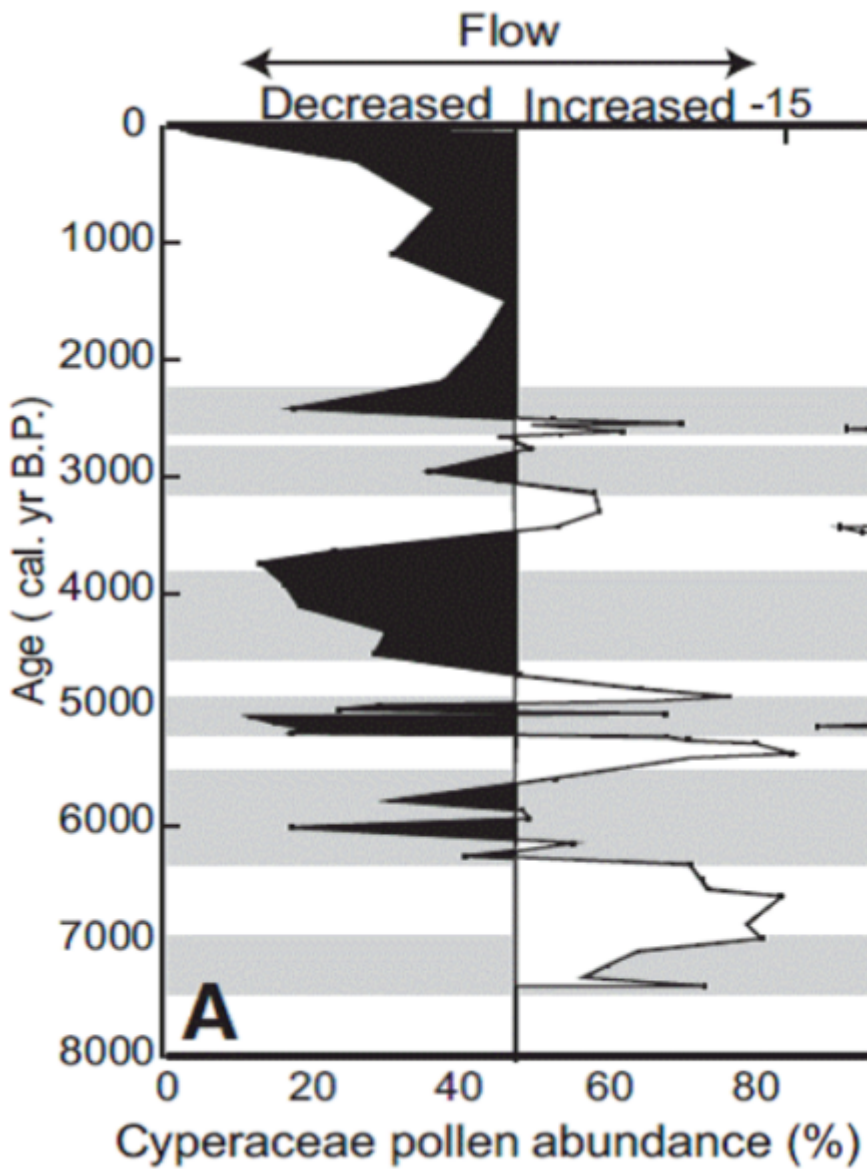
Bild 12.2 [32] Abbildung 1: Dürrephasen im Nileinzugsgebiet markiert durch grau hinterlegte Zonen. Die Wassermenge des Nil war zu diesen Zeiten reduziert (Ausschläge der Kurve nach links), basierend auf Pollen-Analysen. Abbildung aus Bernhardt et al. (2012).
