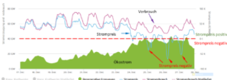
Bild 1 Verlauf von Verbrauch, Strompreis und Ökostromerzeugung vom 17. – 28. Dezember. Quelle: Agorameter
