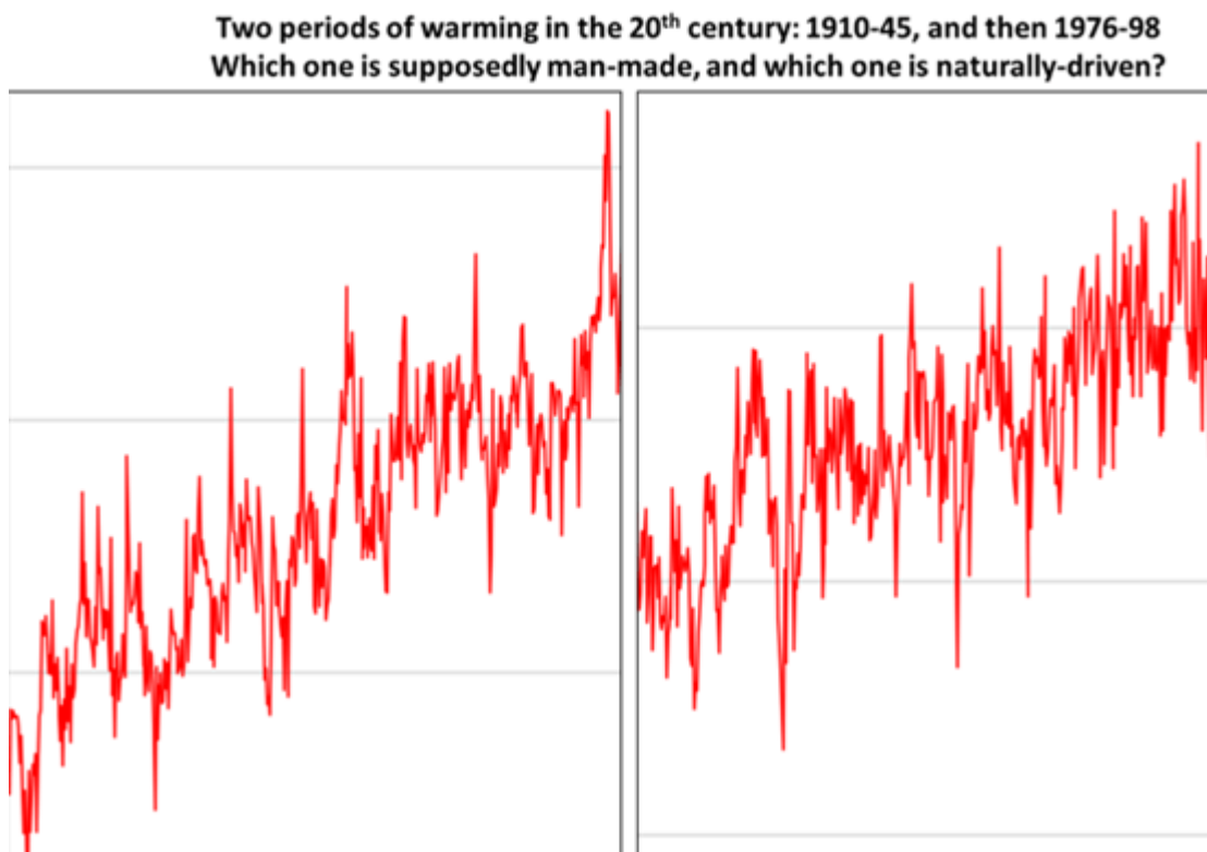
Abbildung 14 – Welcher Temperaturanstieg des 20. Jahrhunderts ist derjenige, der angeblich durch CO 2 -getriebene Erwärmung verursacht wurde?
