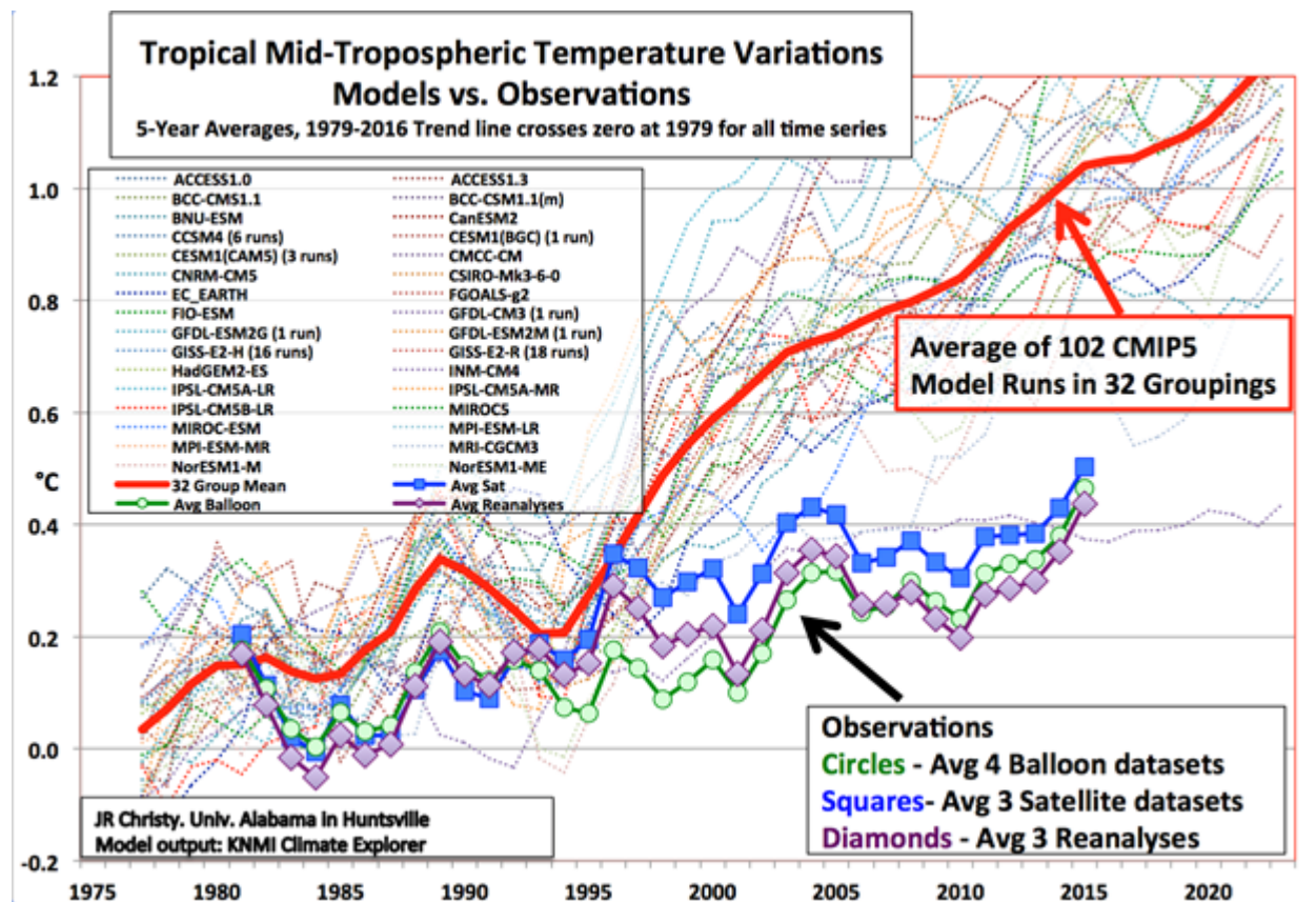
Abbildung 12: Simulation vs. Realität
