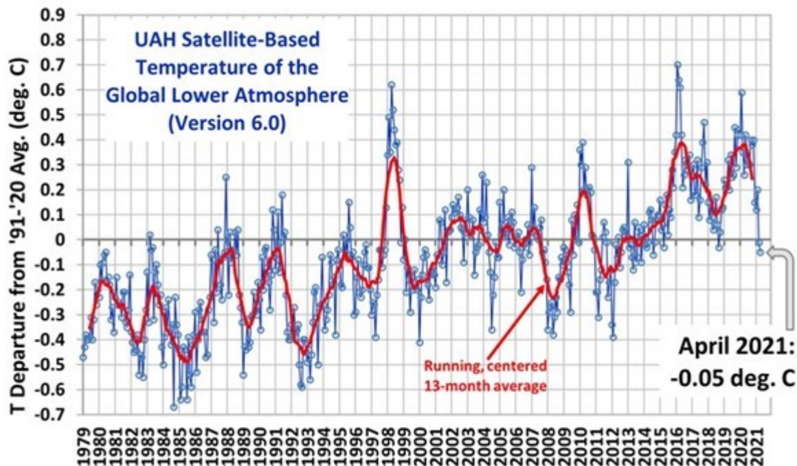
Abbildung 11 – Die neueste Version der MSU-Temperaturen. Diese liegen ungefähr in der 850-300mb Schicht. Quelle
