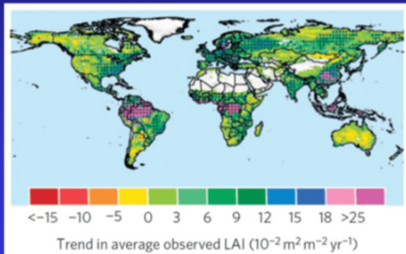
Abbildung 3 – Änderungen des Leaf Area Index , ab 1982
