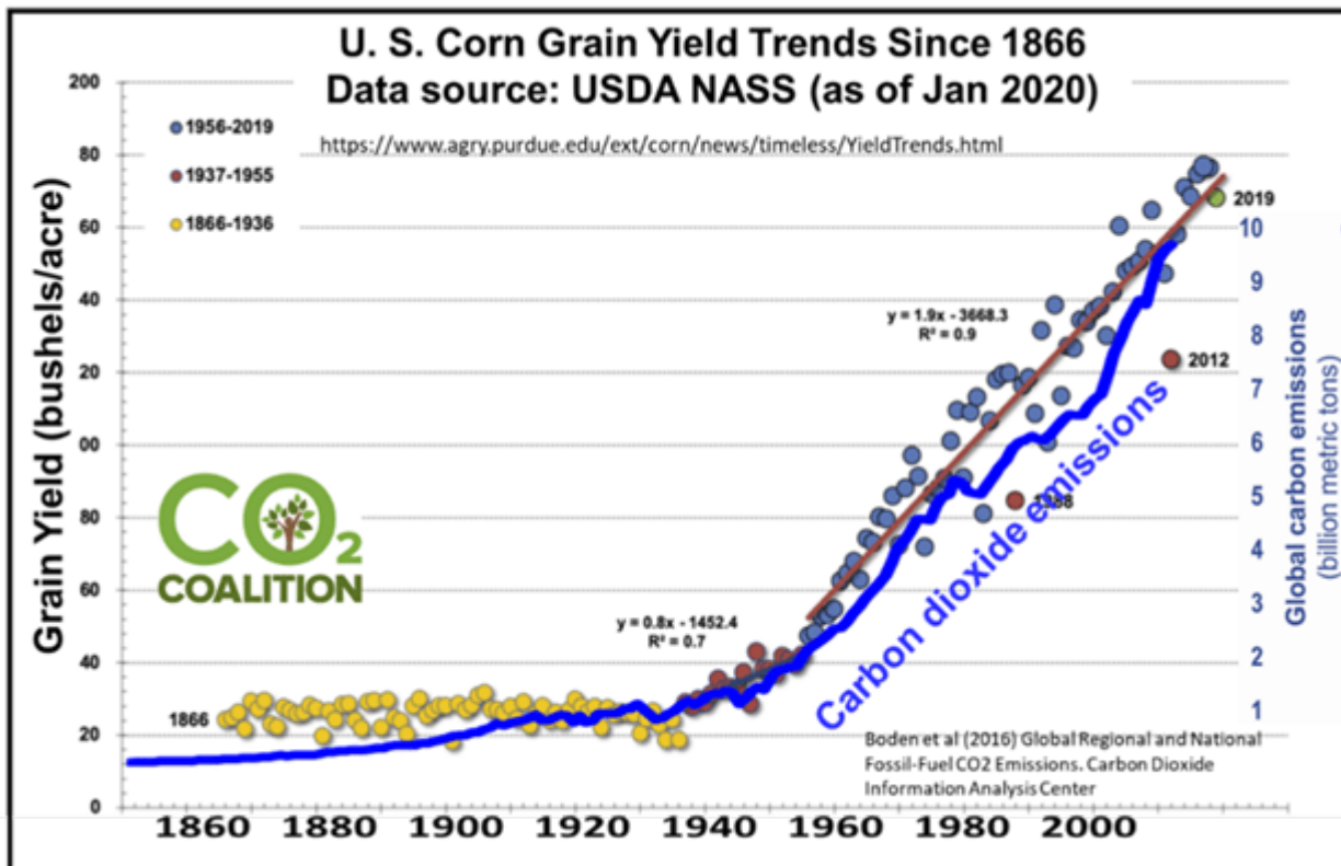
Abbildung 5: Trend der Maisernte in den USA im Vergleich zu globalen Kohlenstoff-Emissionen
