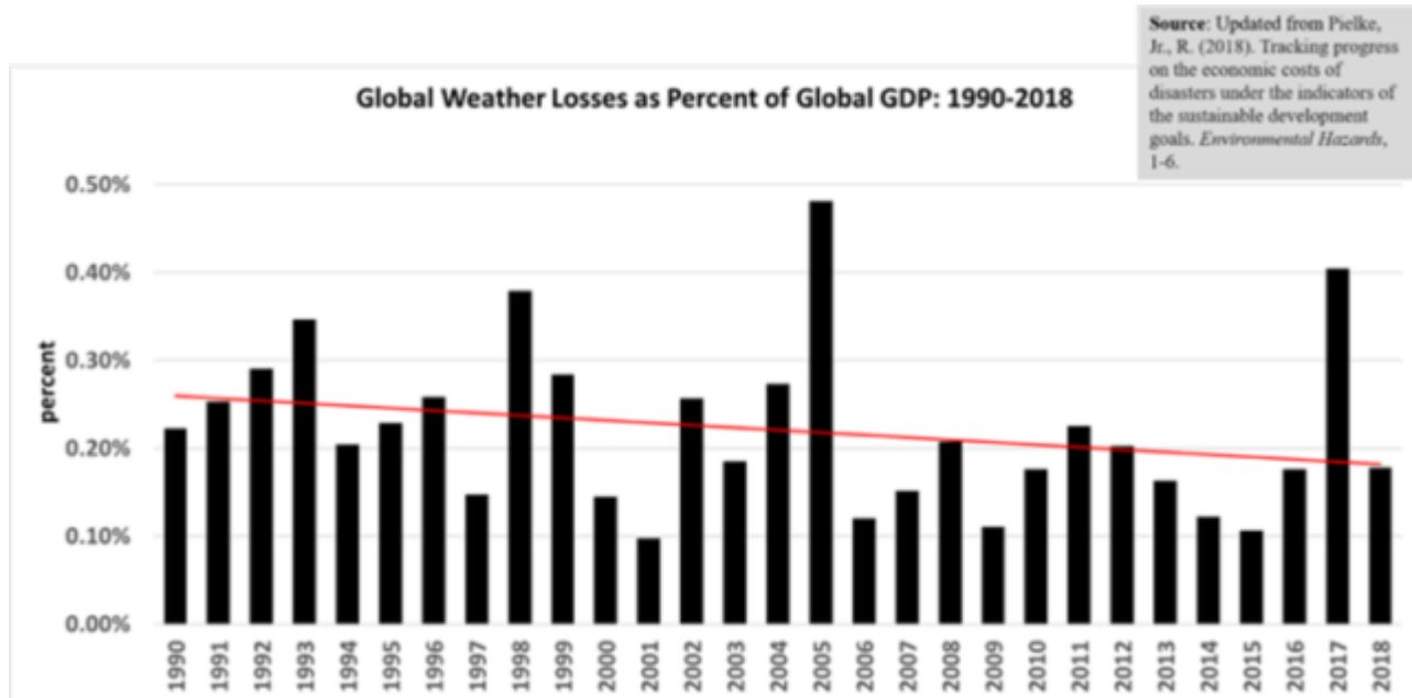
Abbildung 10 – Globale wetterbedingte Schäden in Prozent des globalen BIP bis 2018. Quelle: Pielke, Jr., 2018 update of 2017 paper in Environmental Research.
