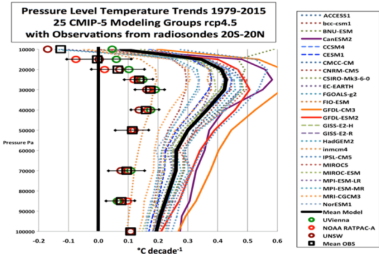
Abbildung 13 – Dicke schwarze Linie: Durchschnittliche Erwärmungstrends pro Dekade. Dünne farbige Linien: Durchschnittliche Erwärmungstrends für jedes Modell. Farbige geometrische Figuren: Beobachtungen. Die vertikale Achse ist die Höhe, gemessen am atmosphärischen Druck. Der maximale Fehler liegt bei 200mb („20000“ in der Grafik). Die durchschnittliche vorhergesagte Erwärmungsrate auf dieser Höhe ist bemerkenswerterweise sechsmal so hoch wie die beobachtete. CMIP-5-Modellfamilie.
