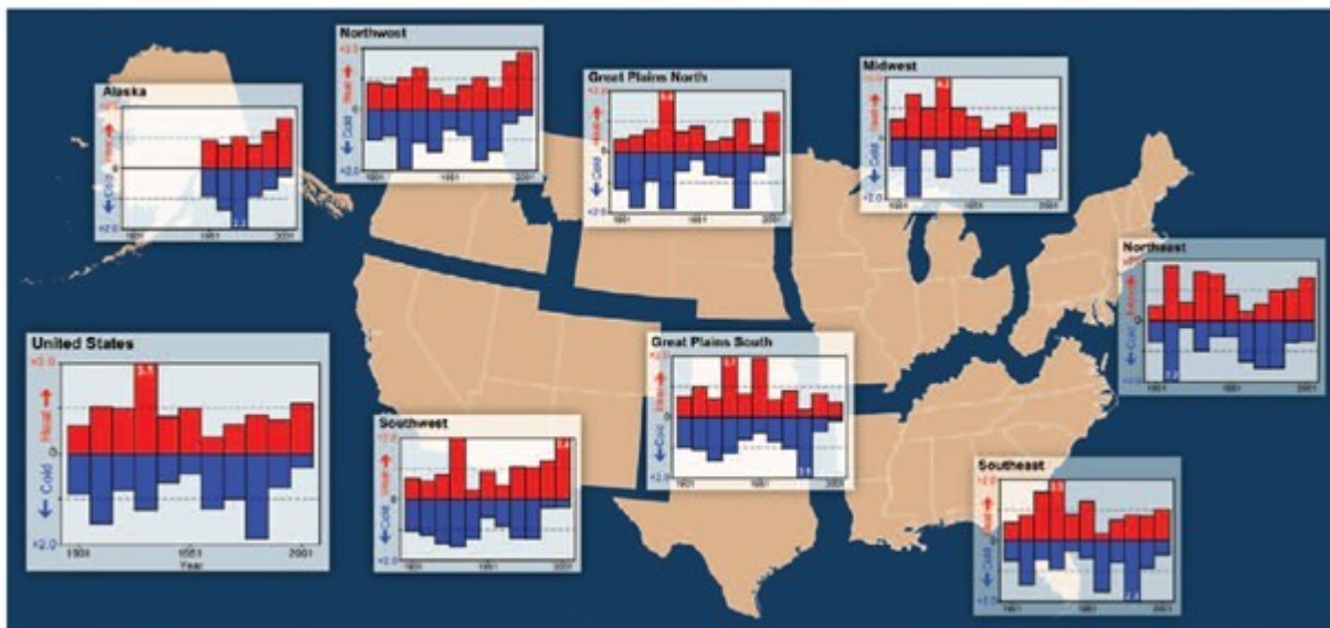
FIG. 1. Time series of decadal-average values of heat wave (red bars) and cold wave (blue bars) indices. These Abbildung 6 – Dekadischer Durchschnitt von Hitzewellen und Kältewellen
