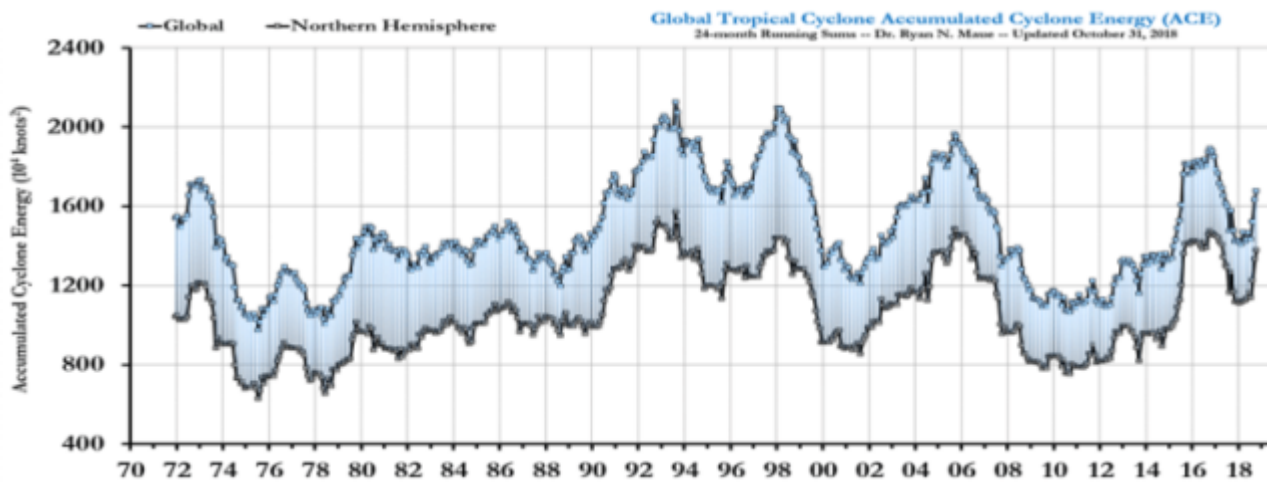
Abbildung 9 – Kumulierte [tropische] Zyklonenergie. Aus Maue, 2011 und Aktualisierungen
