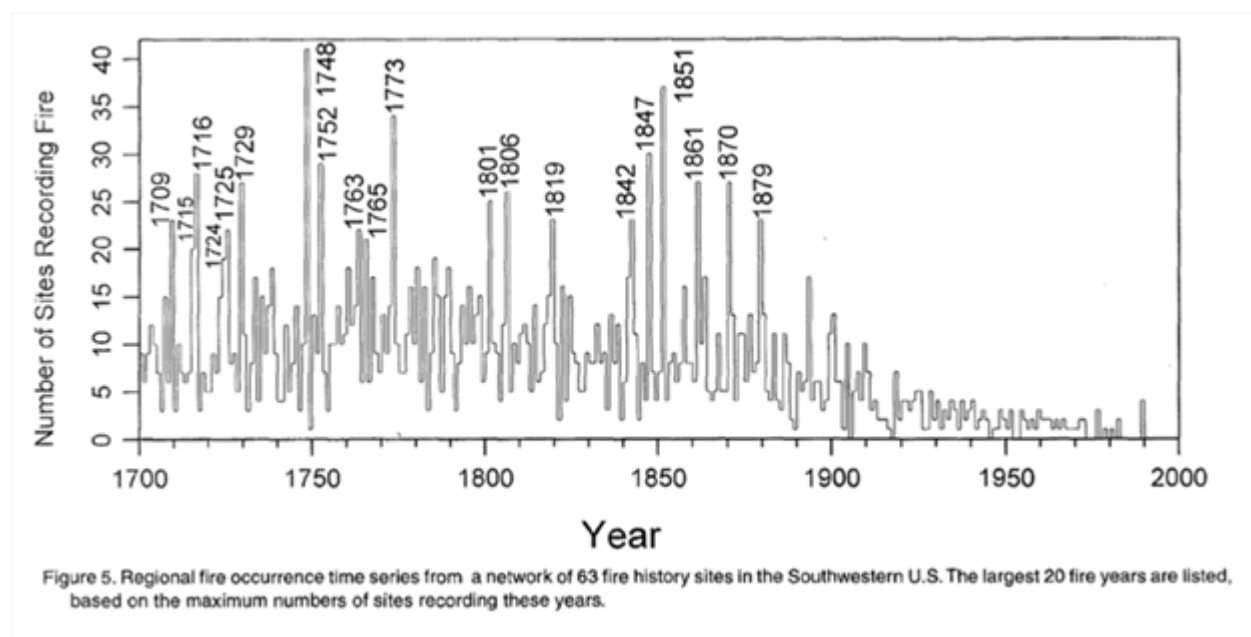
Abbildung 8 – Regionales Auftreten von Bränden über 300 Jahre
