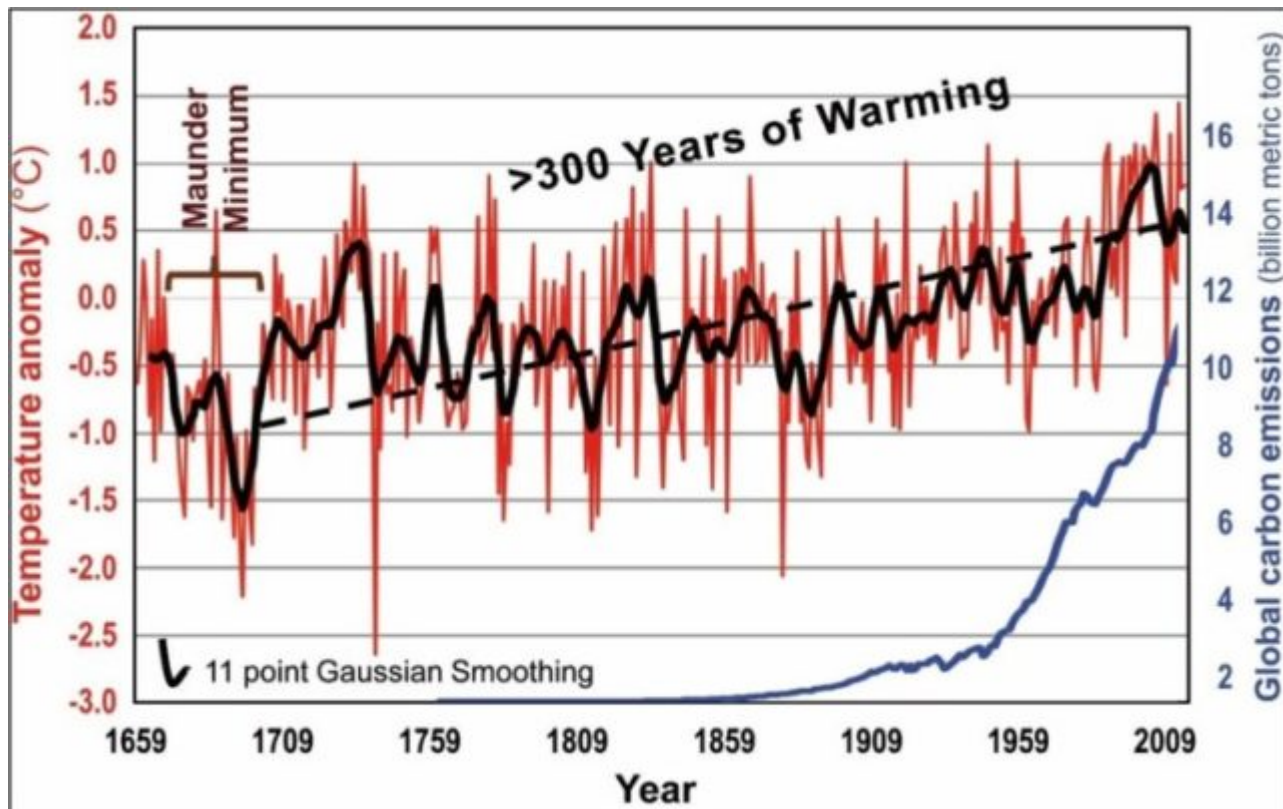
Abbildung 15 – Mehr als 250 Jahre Erwärmung traten auf, bevor der Mensch begann, große Mengen CO 2 in die Atmosphäre einzubringen.
