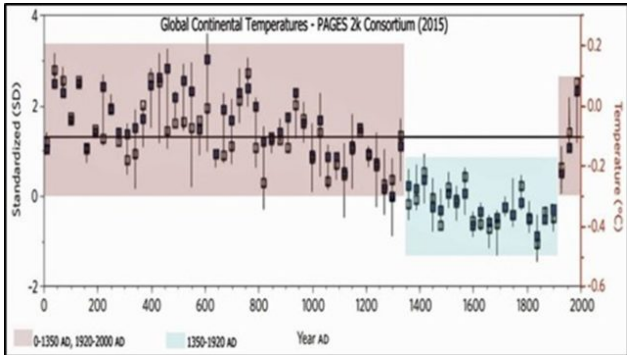
Abbildung 2. Modifiziert aus Gosselin (2018). Quelldaten: Ahmed (2015)
