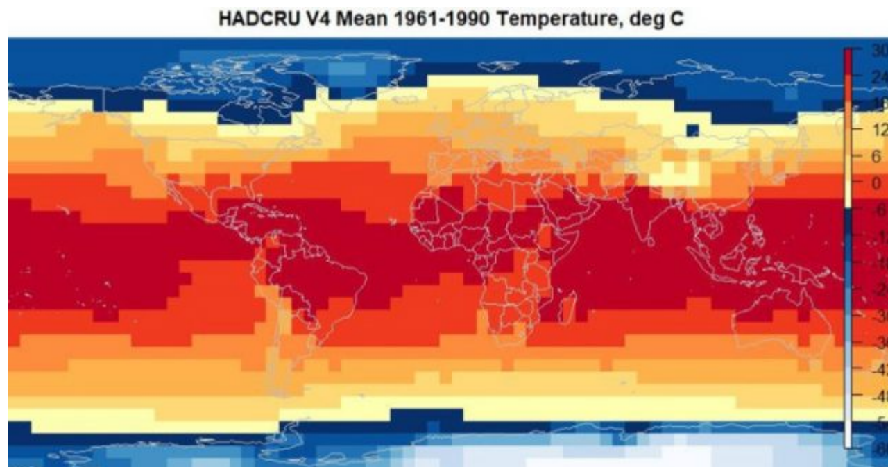
Abbildung 5: Karte der „Absolut“-Daten (Datenquelle: HADCRU )
