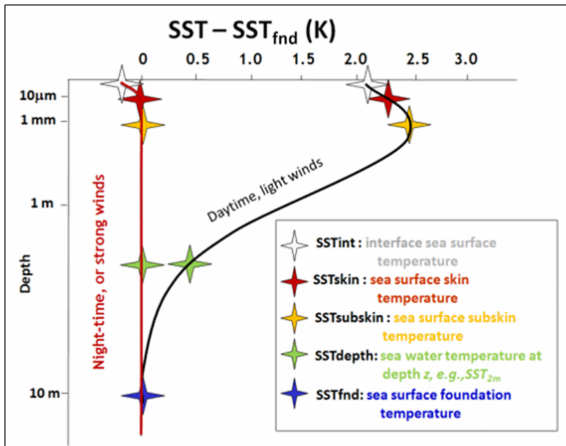
Abbildung 1. Das GHRSSST-Diagramm der Temperatur an der Meeresoberfläche. Die Meeresbedingungen, insbesondere die Windgeschwindigkeit und die Tages- oder Nachtzeit, können einen Unterschied von 2,5 °C oder mehr im Temperaturgradienten von der Oberfläche zur Temperatur des Untergrunds (stabiler Teil der Mischschicht) ausmachen. Die Tiefe bis zum oberen Ende des
