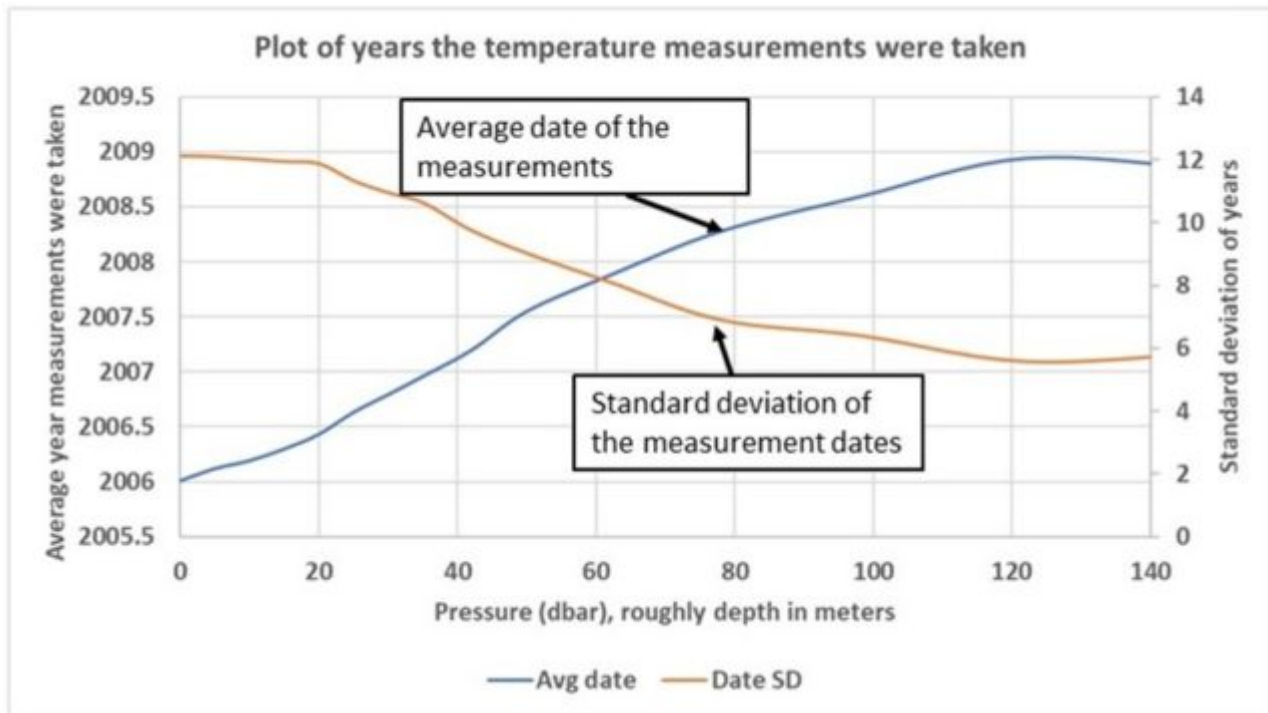
Abbildung 3. Die in Abbildung 2 verwendeten Daten stammen nicht aus einem einzigen Jahr, sondern sind der Durchschnitt der Daten aus über 12 Jahren. Das zentrale Jahr für jede Tiefe ist blau dargestellt (linke Skala) und die Standardabweichung aller verwendeten Jahre ist orange dargestellt (rechte Skala). Datenquelle: Universität Hamburg .
