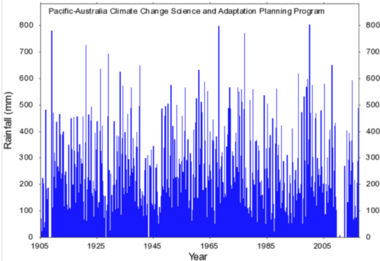
Bild 25 Vanuatu, Port Vila. Monatlicher Niederschlag seit 1905. Quelle: Pacific Climate Change Site Data (bom.gov.au)
