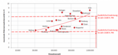
Abbildung 10: Maximale Temperaturerhöhung in Abhängigkeit von der Einwohnerzahl für ausgewählte Städte (beruht auf DWD-Daten von 2010)
