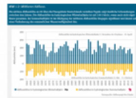
[58] Abfluss: „Nur im Sommer weniger“ Anm.: Aber innerhalb der Schwankungsbreite
