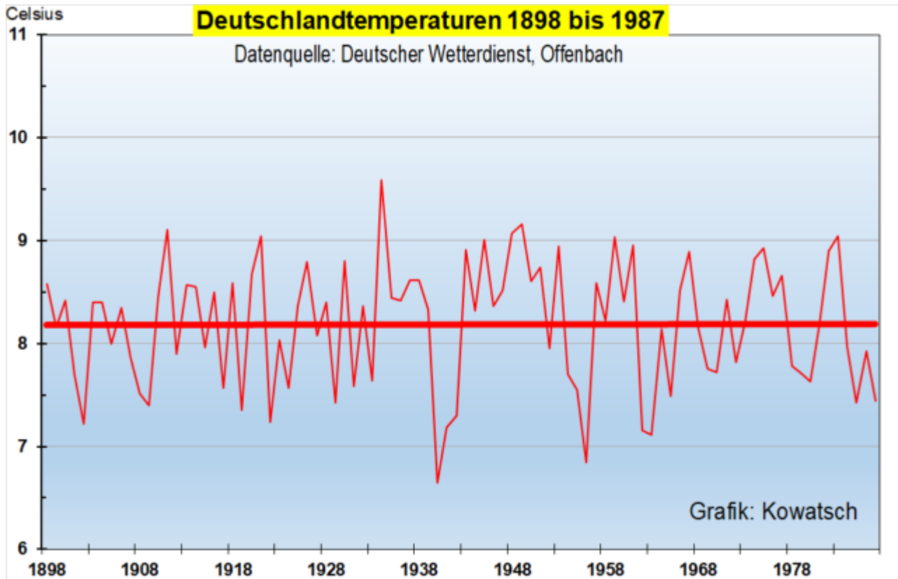
Abb. 2: 90 Jahre lang gab es laut DWD-Temperaturreihe keinerlei Erwärmung in Deutschland, trotz stark steigender \text{CO}_2 -Konzentrationen in der Atmosphäre. Hat die \text{CO}_2 -Erwärmungswirkung etwa 90 Jahre lang ausgesetzt?
