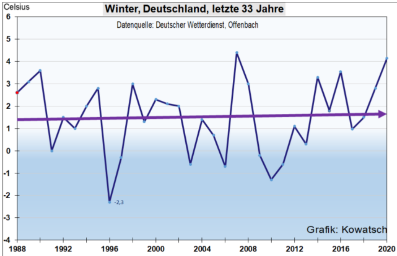
Abb. 7: Die Wintertemperaturen sind seit 1988 in Deutschland nicht weiter angestiegen. Wo ist die Treibhauswirkung des Kohlendioxids im Winter? Antwort: Sie ist nicht existent!
