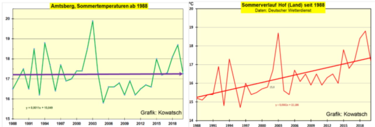
Abb. 6: Wärmeinselarme Stationen zeigen wie alle deutschen Wetterstationen zwar den Temperatursprung 1988, die Temperaturen hielten sich jedoch auf dem milderen Niveau, während die Stationen in wachsenden Wärmeinseln insbesondere im Sommer weiter wärmer wurden. In den letzten Jahren hat die Wetterstation Hof, die seit Jahren in ein Gewerbegebiet eingebaut wird das tiefer liegende und ländliche Amtsberg-Dittersdorf im benachbarten Sachsen überholt.
