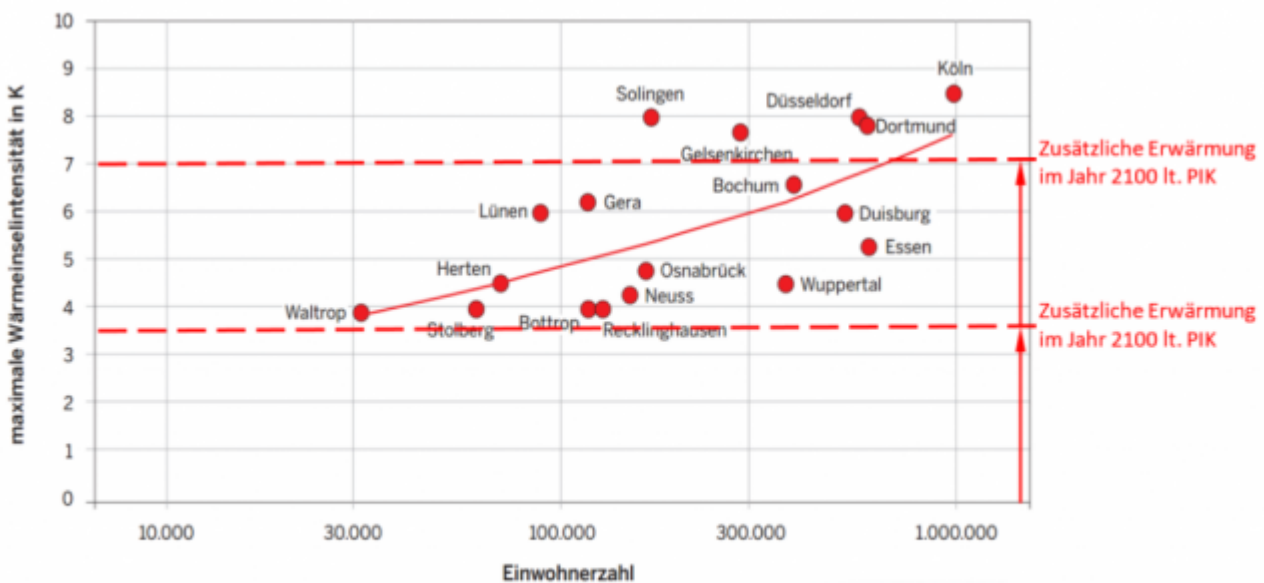
Abbildung 32: Maximale Wärmeinselintensitäten in Abhängigkeit von der Einwohnerzahl für ausgewählte Städte überwiegend aus NRW (KUTTLER 2011)
