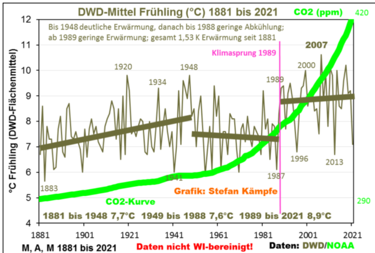
Abbildung 1: Bei den Frühlingstemperaturen in Deutschland sind drei Entwicklungsphasen erkennbar: Eine merkliche Erwärmung um 1,1 K bis 1948, danach eine geringe Abkühlungsphase bis 1988 trotz stark steigender CO 2 -Konzentrationen; ab 1989 ein Klimasprung mit gehäuft sehr warmen Lenzen, gipfelnd in 2007 bei nur noch unwesentlicher Erwärmung. Diese DWD-Daten sind nicht WI-bereinigt; andernfalls wäre die Erwärmung geringer ausgefallen.
