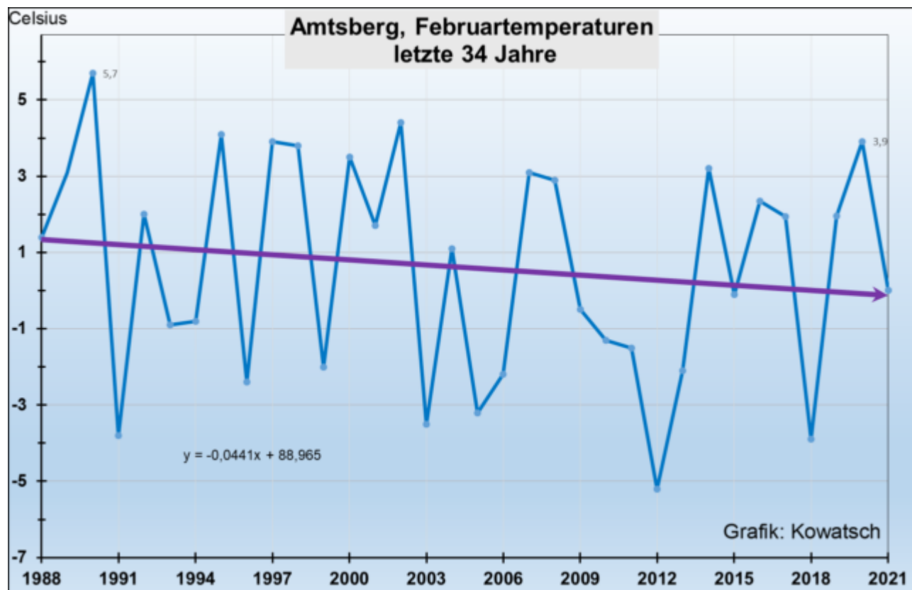
Abbildung 7: Die Wetterstation in einem Vorort von Amtsberg am Fuße des Erzgebirges steht in einem großen Garten am Ortsrand. Die Trendlinie zeigt seit 1988 eine kräftigere Abkühlung als die DWD-
