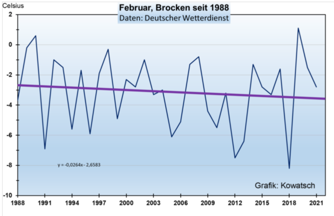
Abbildung 9: Die Wetterstation auf dem 1142 m hohen Brocken zeigt eine stärkere Februarabkühlung in den letzten 34 Jahren als das DWD-Flächenmittel. So ähnlich verhalten sich fast alle höheren Bergstationen
