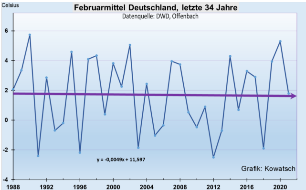
Abbildung 5: Von 1986 auf 1988 erreichte der Februar mit einem Temperatursprung ein höheres Wärmeniveau, seitdem kühlte er trotz Wärmeinseleffektzunahme der DWD-Wetterstationen und starkem CO 2 -Konzentrationsanstieg minimal ab.
