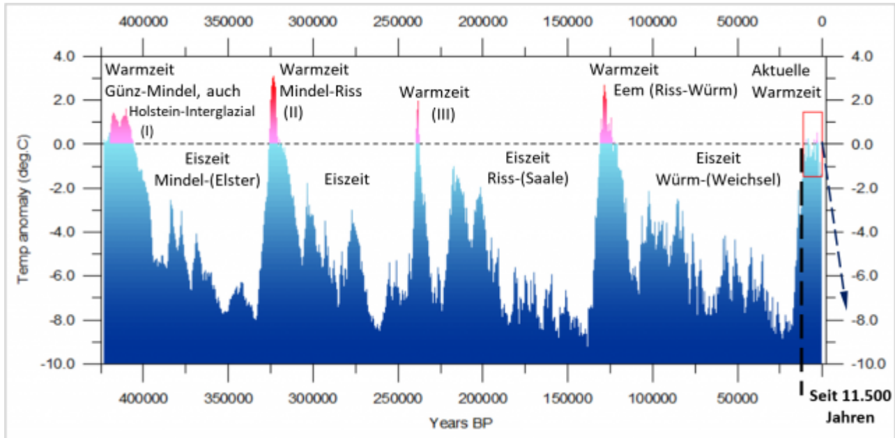
Bild 3 [4] Temperaturverlauf der letzten 450.000 Jahre. Quelle: www.climate4you.com – Ole Humlum – Professor, University of Oslo Department of Geosciences. Vom Autor um Angaben zu den letzten vier Eiszeiten der Alpen ergänzt
