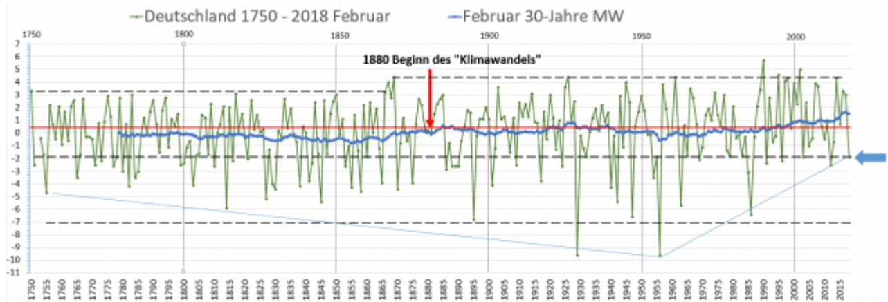
Bild 2 Langzeit-Temperaturreihe Deutschland 1750 – 2018, Februar.
