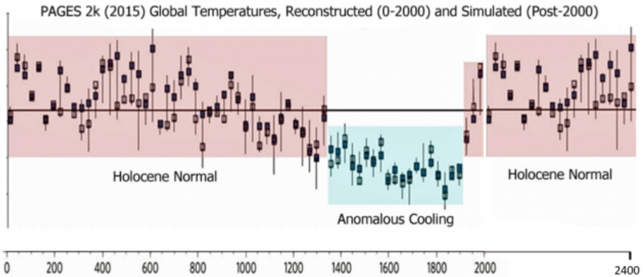
Bild 4 Neue Langzeitrekonstruktion der Globaltemperatur vom Jahr 0 bis 2400 [3]. Vom Autor mit dem Jahr 2400 ergänzt Im Bild 4 ist es nicht so deutlich sichtbar, in einem Bild (Bild 5) aus dem letzten IPCC-Bericht sieht man es aber genau: Die „AGW“-Erwärmung begann bereits weit vor der Industrialisierung, irgendwann um 1600, nicht erst ab 1880 (wie man es angeblich im Welt-Klimavertrag annimmt, obwohl dort keine Zahl erscheint).
