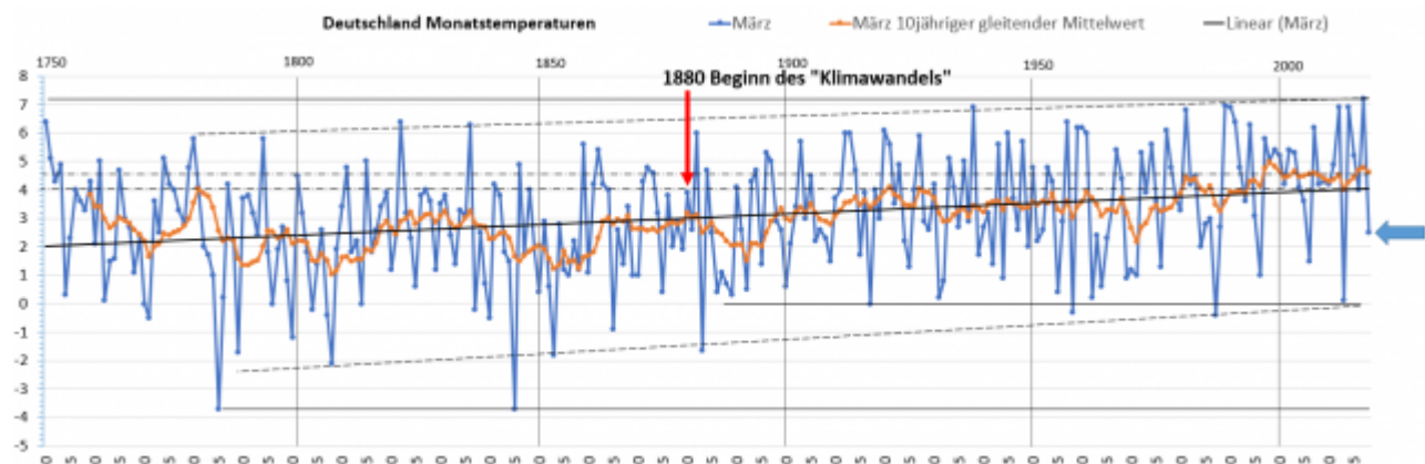
Bild 1 Langzeit-Temperaturreihe Deutschland 1750 – 2018, März. Quelle: WIKIPEDIA (DWD)
