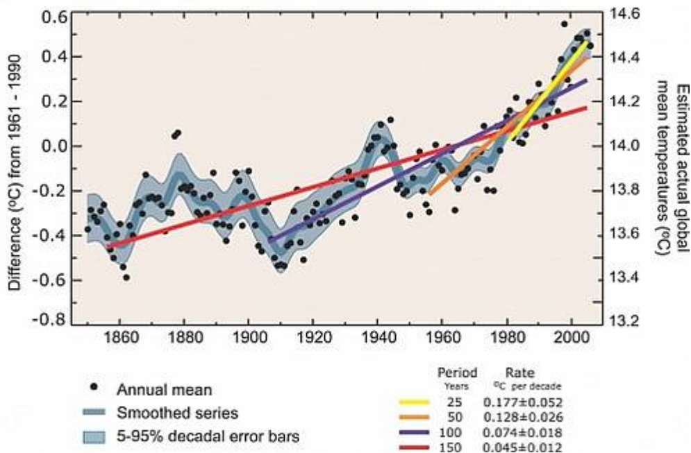
IPCC-Schwindelgraphik mit vier Temperaturtrendlinien
