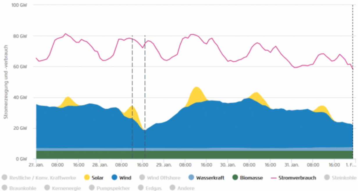
Bild 6 Ganglinien 27.01. – 31.01.2016. Zeitraum 27.01., 12 – 17 h gekennzeichnet. Quelle Agora Viewer
