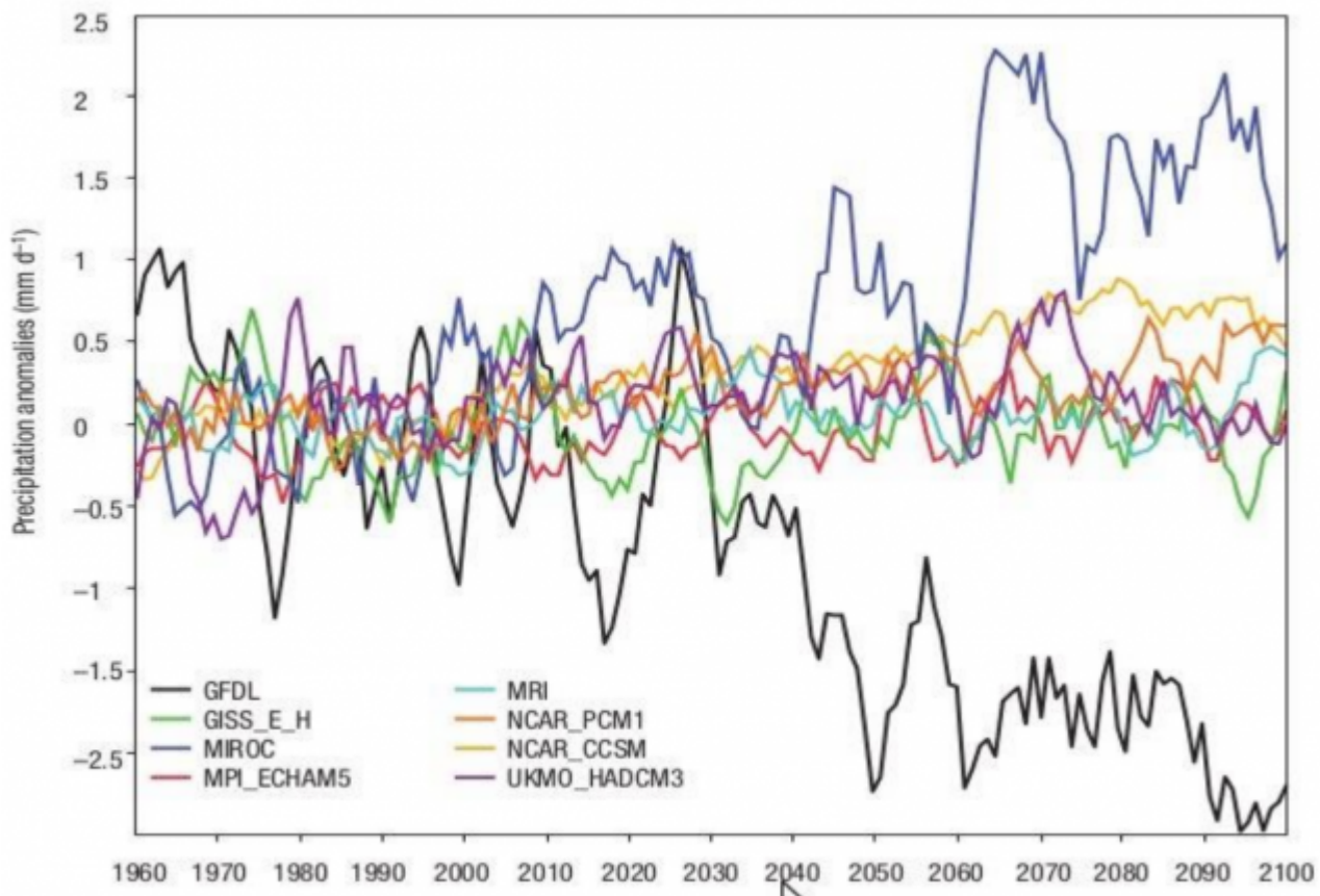
Bild 9 Darstellung aus der Studie mit den Ergebnissen verschiedener Projektions-Testläufe. [16] Figure 1.7: The JAS-mean Sahel rainfall anomalies from CMIP3 models. This figure is from Cook 2008 ('News & Views' in Nature).
