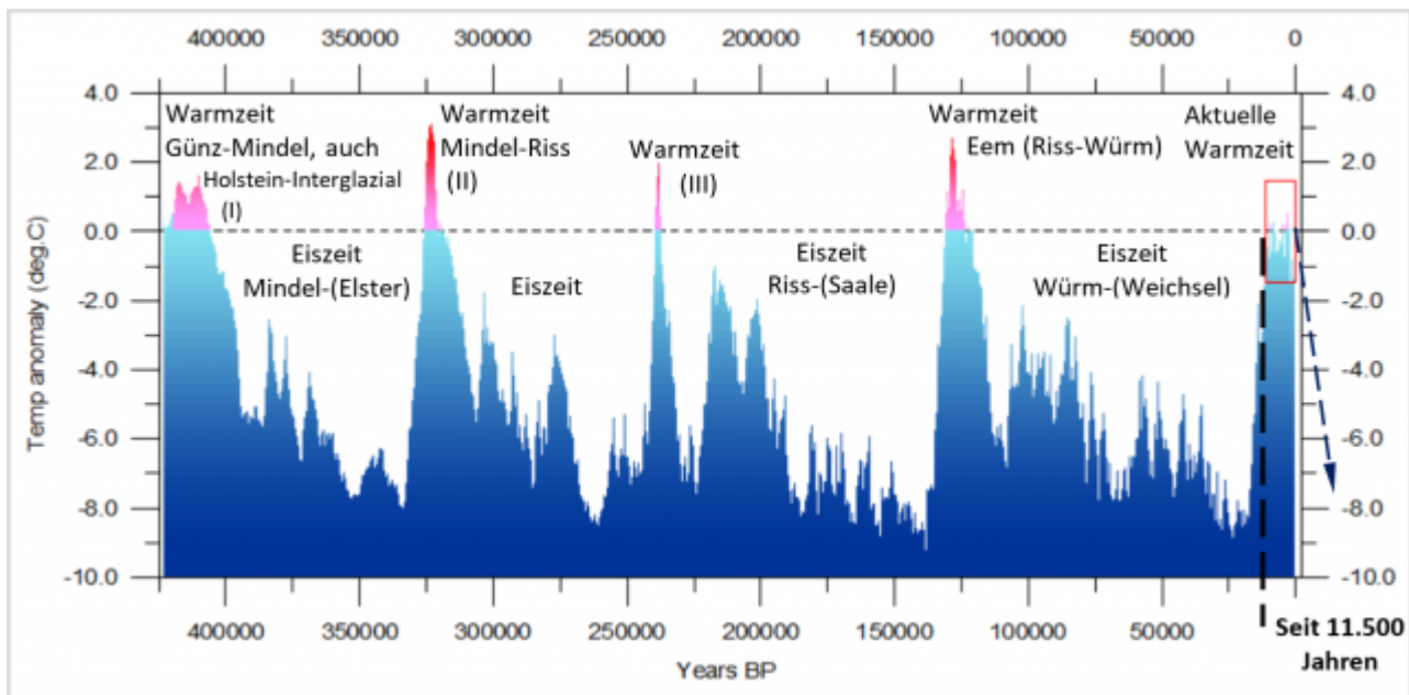
Bild 7 [18] Temperaturverlauf der letzten 450.000 Jahre. Quelle: climate4you.com – Ole Humlum – Professor, University of Oslo Department of Geosciences. Vom Autor um Angaben zu den letzten vier Eiszeiten der Alpen ergänzt
