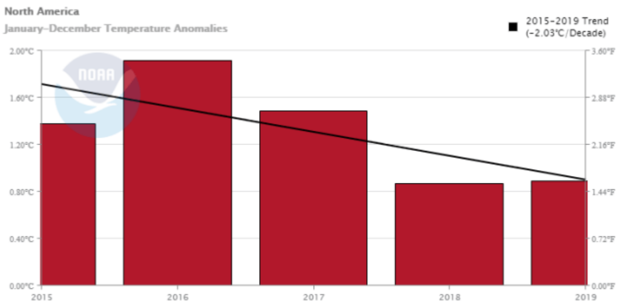
Abbildung E1: Nordamerika, Abkühlung um 2,03^{\circ}\text{C} pro Dekade. Quelle
