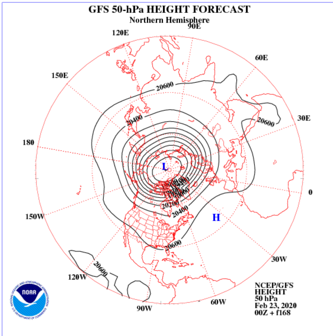
Abbildung 1: Klassisch ausgeprägter Stratosphärischer Polarwirbel, hier im 50-hPa-Niveau (ca. 20 km Höhe), und zwar als numerische Simulation über eine Woche im Voraus. Quelle: NOAA
