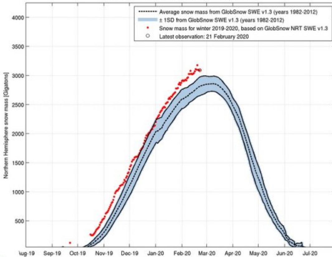
Abbildung 8: Volumen der winterlichen Schneemenge. Quelle
