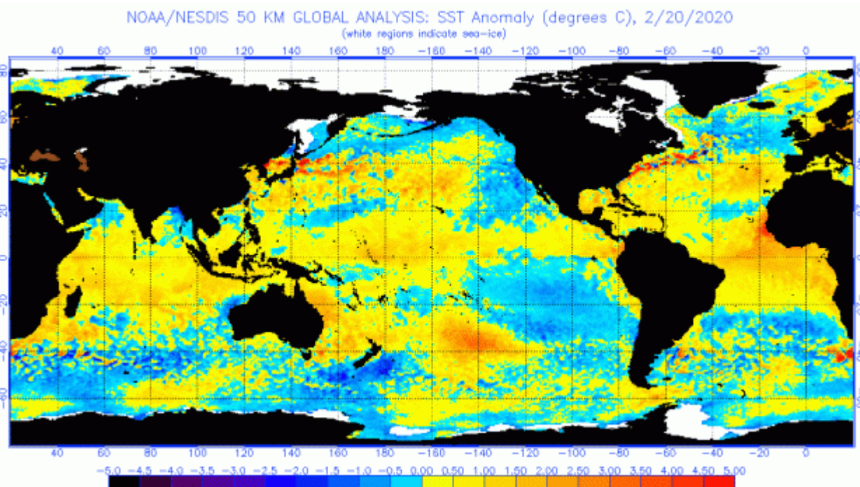
Abbildung 12: Wassertemperatur-Anomalien, 20. Februar 2020. Man erkennt die deutliche Abkühlung im Nordatlantik. Quelle
