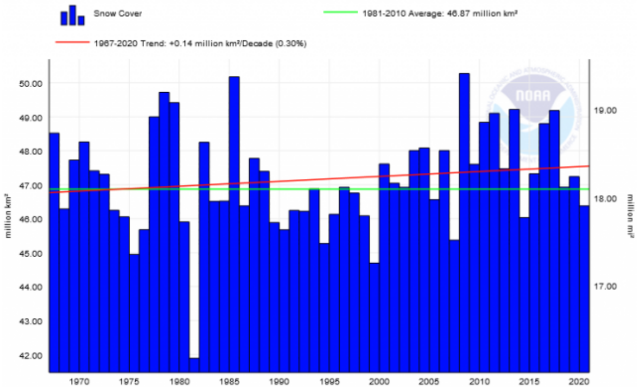
Abbildung 7: Überraschung: Es zeigt sich neben der üblichen Variation eher ein steigender Trend! Quelle
