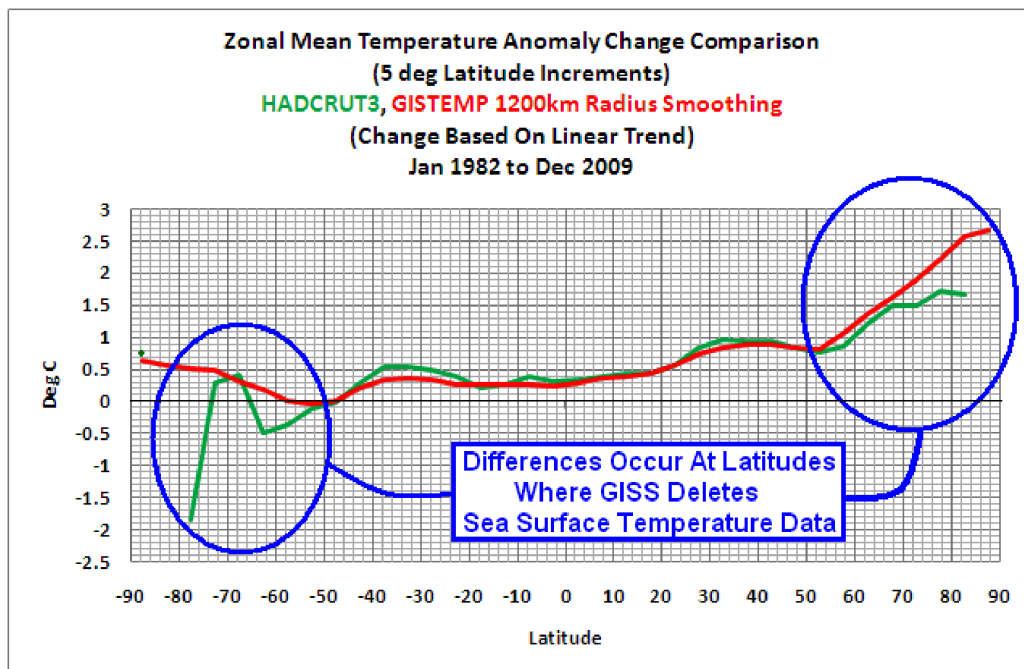
Abb. 10 Vergleich der mittleren zonalen Temperaturanomalie für Segmente von 5° geogr. Breite GISTEMP mit 1200-km-Radius minus HADCRUT3 (Änderungen basierend auf dem linearen Trend) Jan 1982 bis Dez. 2009 Unterschiede zeigen sich dort, wo GISS Wassertemperaturen wegfällen lässt
