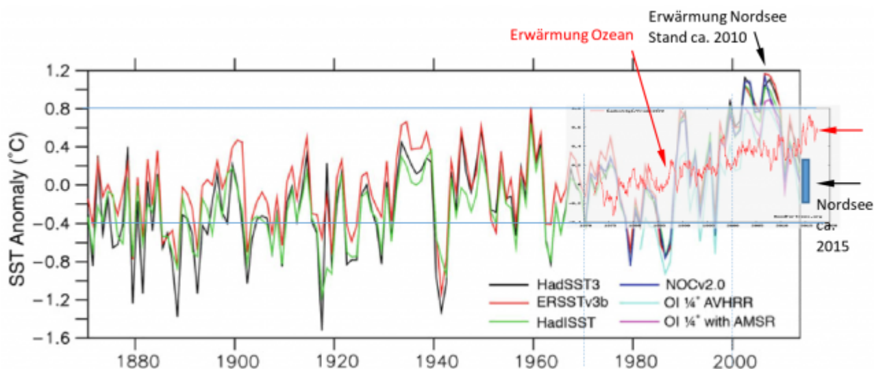
Bild 3 [2] Fig. 3.3 North Sea region annual sea-surface temperature (SST) anomalies relative to the 1971–2000 average. Darüber gelegt die HadSST3-Temperaturen Ozean. Quelle: Woodfortrees
