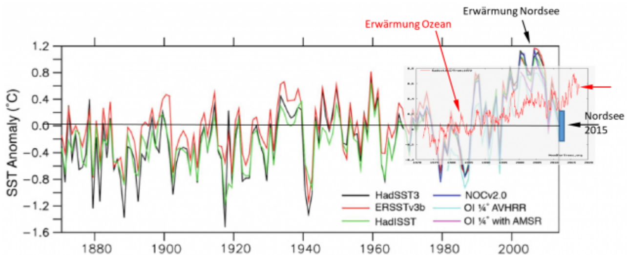
Bild 4 Phasenverschiebung der Erwärmungen von Bild x angepasst
