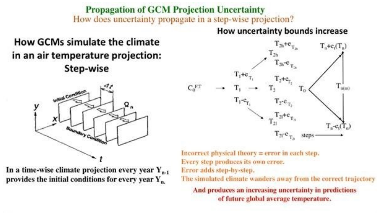
Abbildung 3: Zunahme der Unsicherheit einer Projektion der Lufttemperatur. C_0^{F,T} ist der Grundzustand des Klimas, welcher einen initialen Antrieb F_0 aufweist, der Null sein kann, und eine initiale Temperatur T_0 . Die finale Temperatur T_n wird festgelegt durch die finale Unsicherheit \pm e_t als T_n \pm e_t .
