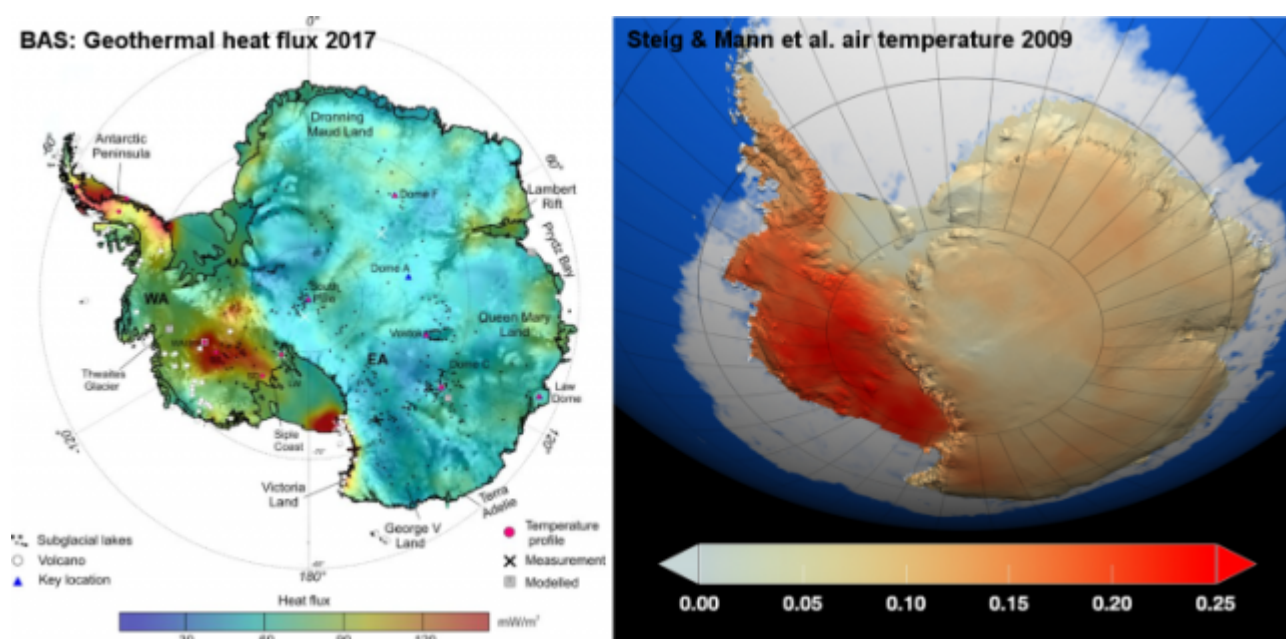
Abbildung 4: Vergleich des geothermischen Flusses (links) mit dem Trend der Temperatur-Anomalie von Steig et al. 2009 in Grad Celsius (rechts). Graphischer Vergleich erstellt von Anthony Watts.
