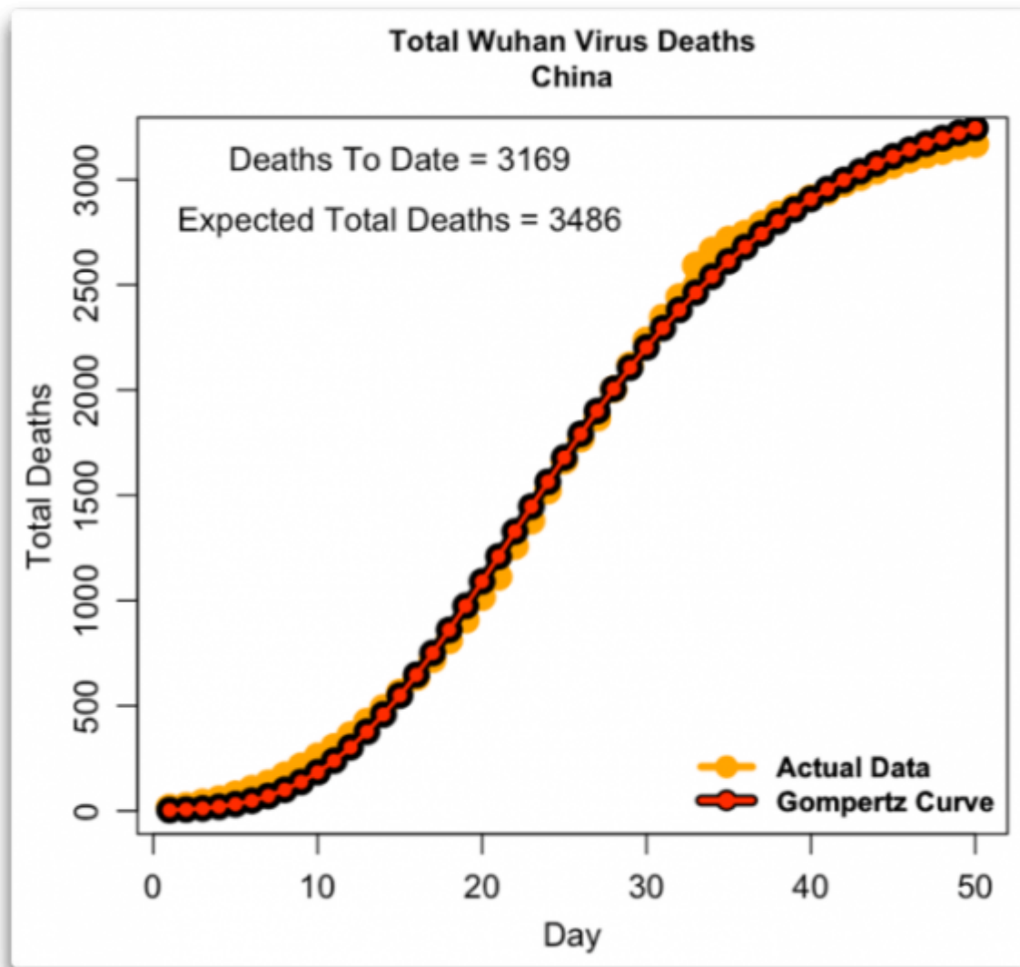
Abbildung 5: Gesamtzahl der Todesfälle durch das Corona-Virus in China, zusammen mit einer Best Fit -Gompertz-Kurve der Daten.
