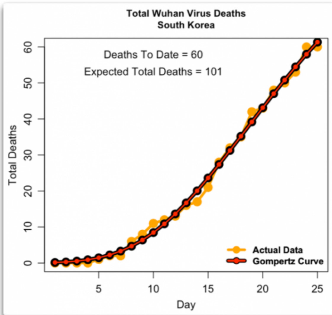
Abbildung 6: Gesamtzahl der Todesfälle durch das Corona-Virus, wieder mit dem Best Fit einer Gompertz-Kurve für die Daten.
