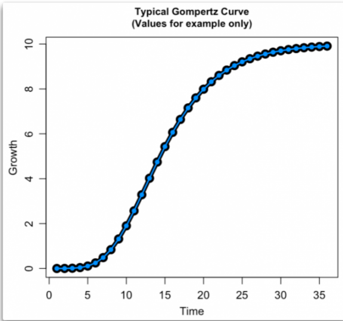
Abbildung 3: Eine typische Gompertz-Kurve, welche die Entwicklung der Anzahl der Gesamtfälle oder die Gesamtzahl der Todesfälle während einer Epidemie zeigt.
