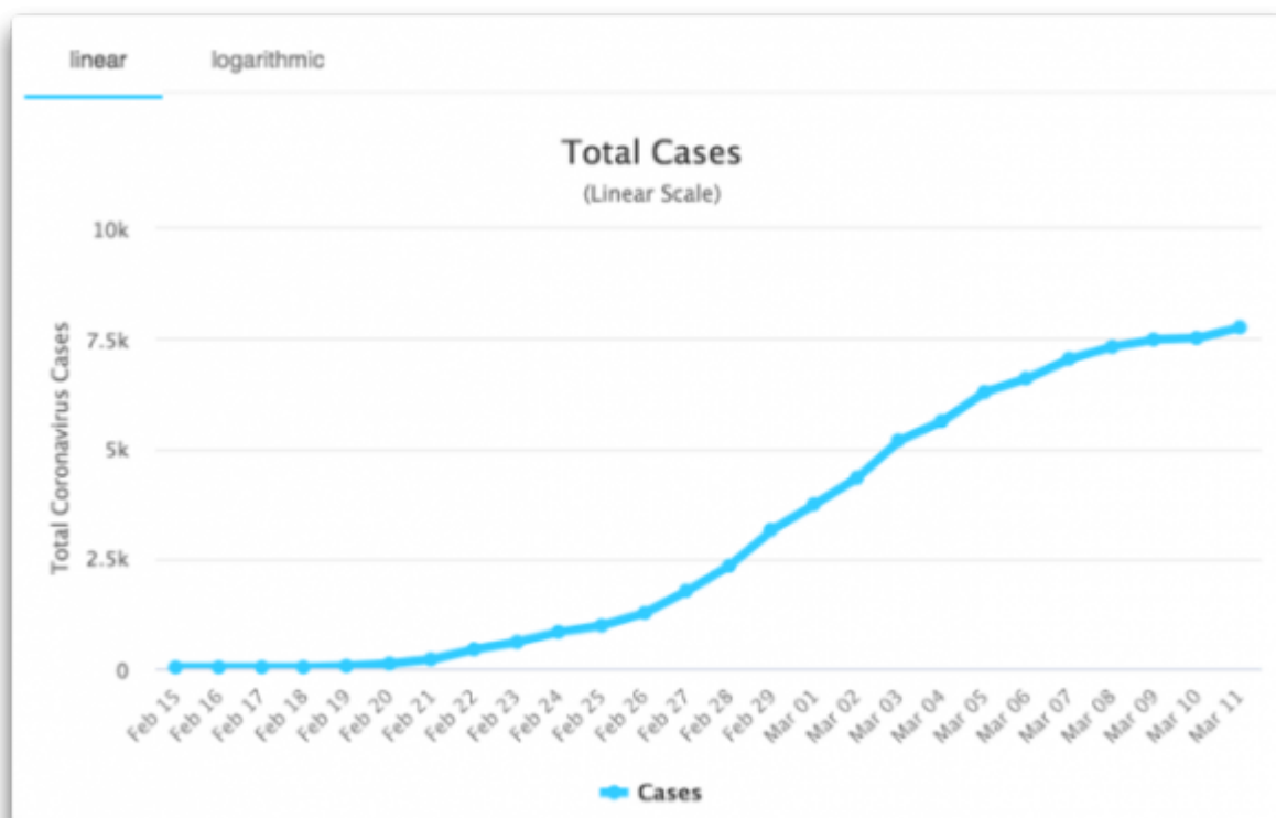
Abbildung 1: Gesamtzahl der Coronavirus-Fälle seit Beginn der Epidemie. Quelle
