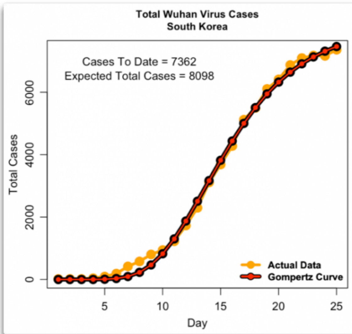
Abbildung 4: Gesamtzahl der Corona-Fälle in Südkorea, zusammen mit der Best Fit -Gompertz-Kurve für die Daten.
