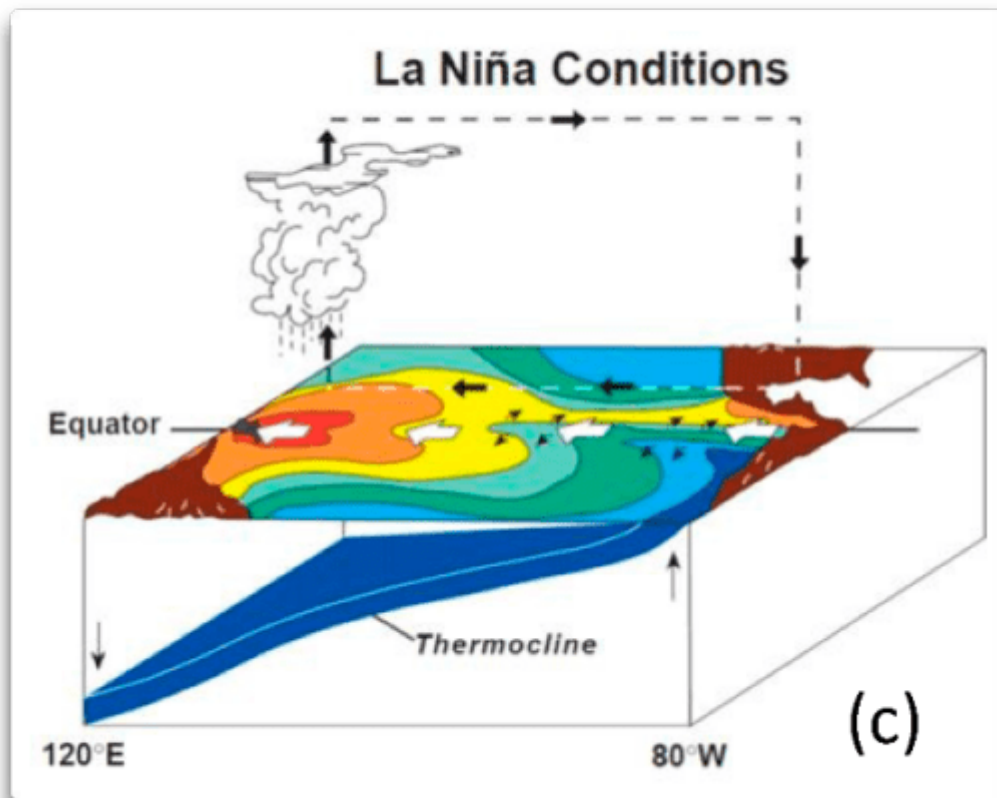
Abbildung 6: Schematische Darstellung der La Nina-Bedingungen
