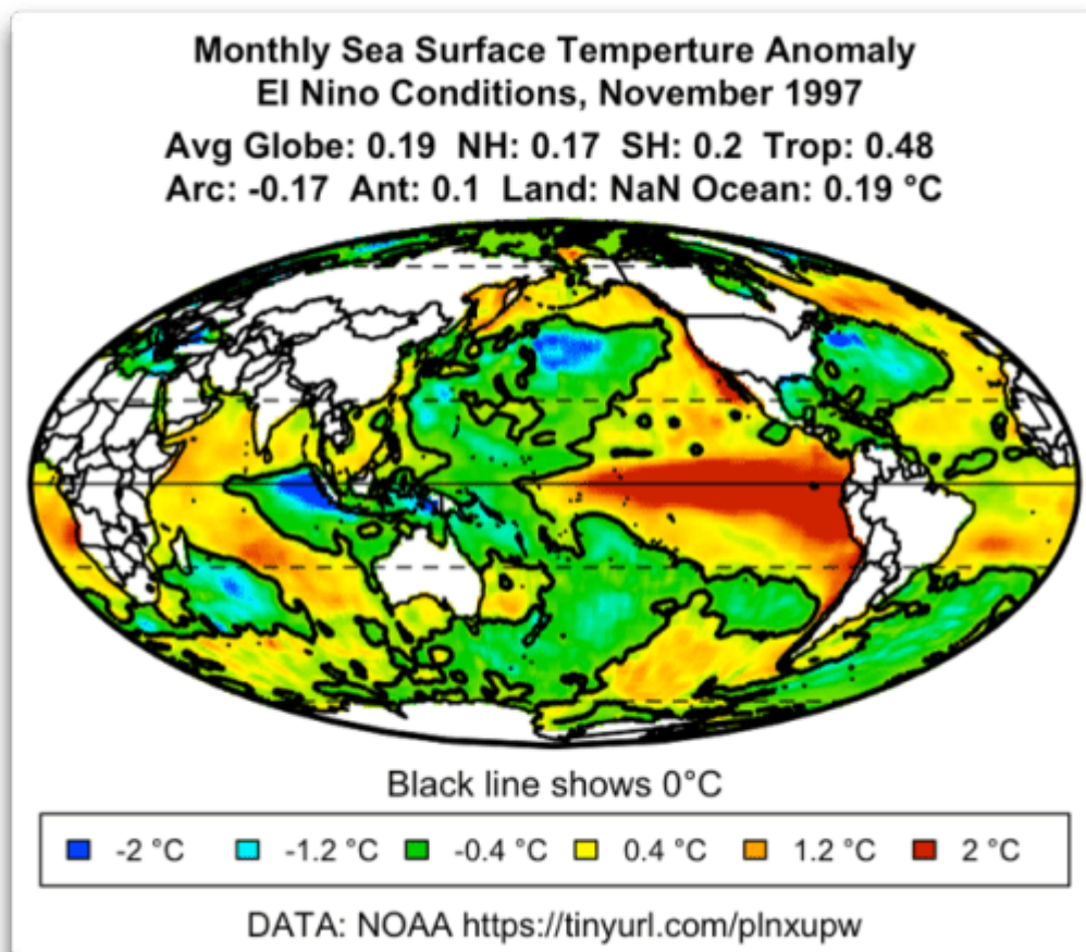
Abbildung 5: Anomalie der Meeresoberflächentemperatur (jahreszeitliche Schwankungen beseitigt) während des Höhepunktes (November) des großen El Nino von 1997-1998. Dies zeigt den großen Hitzestau entlang des Äquators im östlichen Pazifik in der Nähe des amerikanischen Kontinents.
