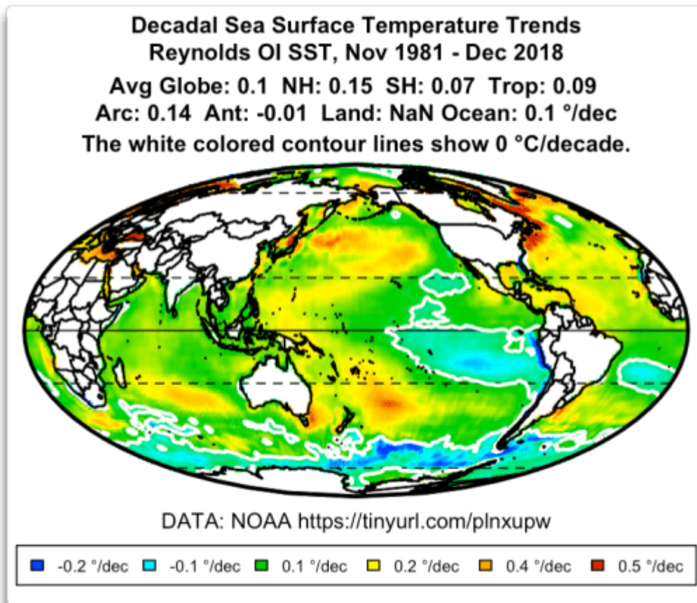
Abbildung 12: Dekadische Trends der Meeresoberflächentemperatur.
