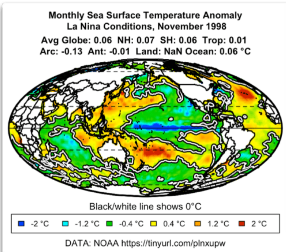
Abbildung 8: Abbildung 8. SST-Anomalie (saisonale Schwankungen entfernt) während eines La Nina-Höhepunktes.
