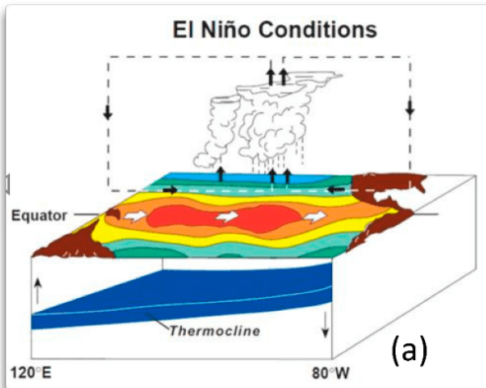
Abbildung 3: El Niño-Bedingungen. Die Oberfläche in der Nähe von Amerika ist wärmer. Die Sprungschicht vor der Küste Amerikas ist tiefer.
