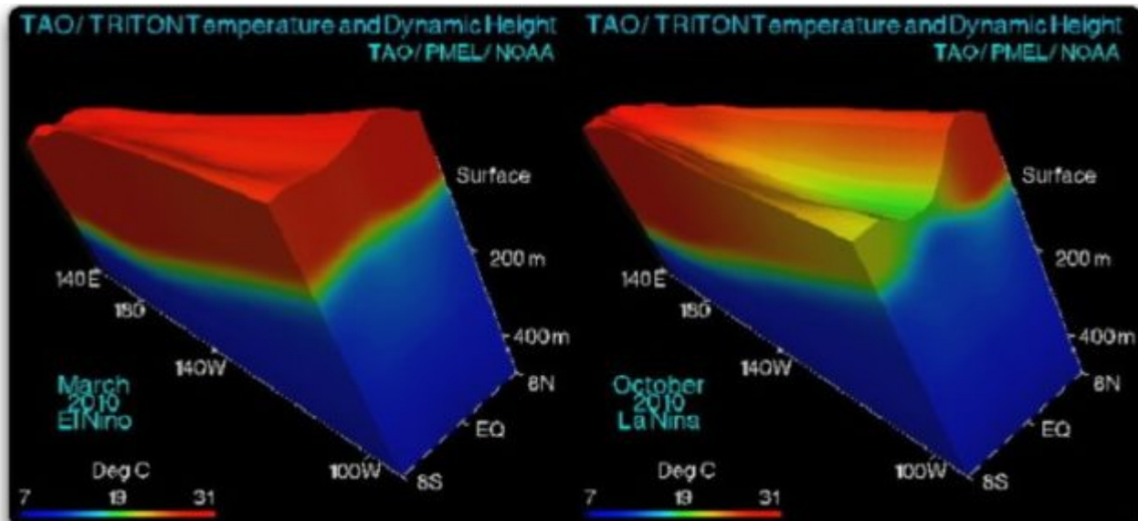
Abbildung 9: Die Nino/Nina-Unterschiede, wie sie durch die TAU/TRITON vertäuten Bojen entlang des Äquators gezeigt werden. Sie blicken nach Westen, über den Äquator im Pazifik, von einem Aussichtspunkt irgendwo in den Anden in Südamerika. Die farbigen Flächen zeigen die Meerestemperaturen von TAO/TRITON. Die obere Fläche ist die Meeresoberfläche, von 8°N bis 8°S und von 137°E bis 95°W. Die Form der Meeresoberfläche wird durch TAO/TRITON Dynamic Height-Daten bestimmt. Die breite vertikale Oberfläche liegt bei 8°S und erstreckt sich bis in 500 Meter Tiefe. Die schmalere vertikale Oberfläche befindet sich bei 95°W. Alle diese Daten stammen von der TAO/TRITON-Anordnung vertäuter Ozeanbojen im äquatorialen Pazifik.
