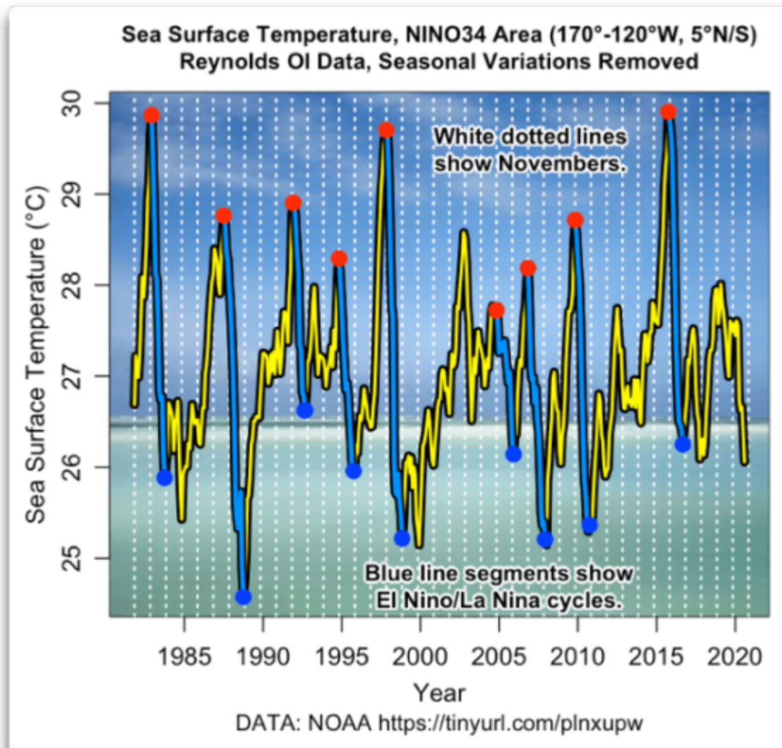
Abbildung 11. Meeresoberflächentemperatur im NINO34-Gebiet. Blaue Abschnitte zeigen die Zeiten, zu denen der Pumpvorgang stattfindet. Rote Punkte zeigen die Spitzenwerte der El Nino-Bedingungen und blaue Punkte die Spitzenwerte der La Nina-Bedingungen. Gepunktete vertikale weiße Linien zeigen den November eines jeden Jahres.
