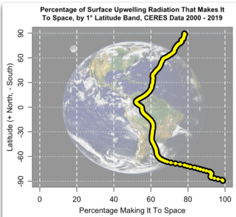
Abbildung 10: Abbildung 10. Menge der aufsteigenden Oberflächenstrahlung, die es in den Weltraum schafft, in einem Breitenband von 1°. Dies sind Monatsdurchschnitte über den gesamten Aufzeichnungszeitraum.
