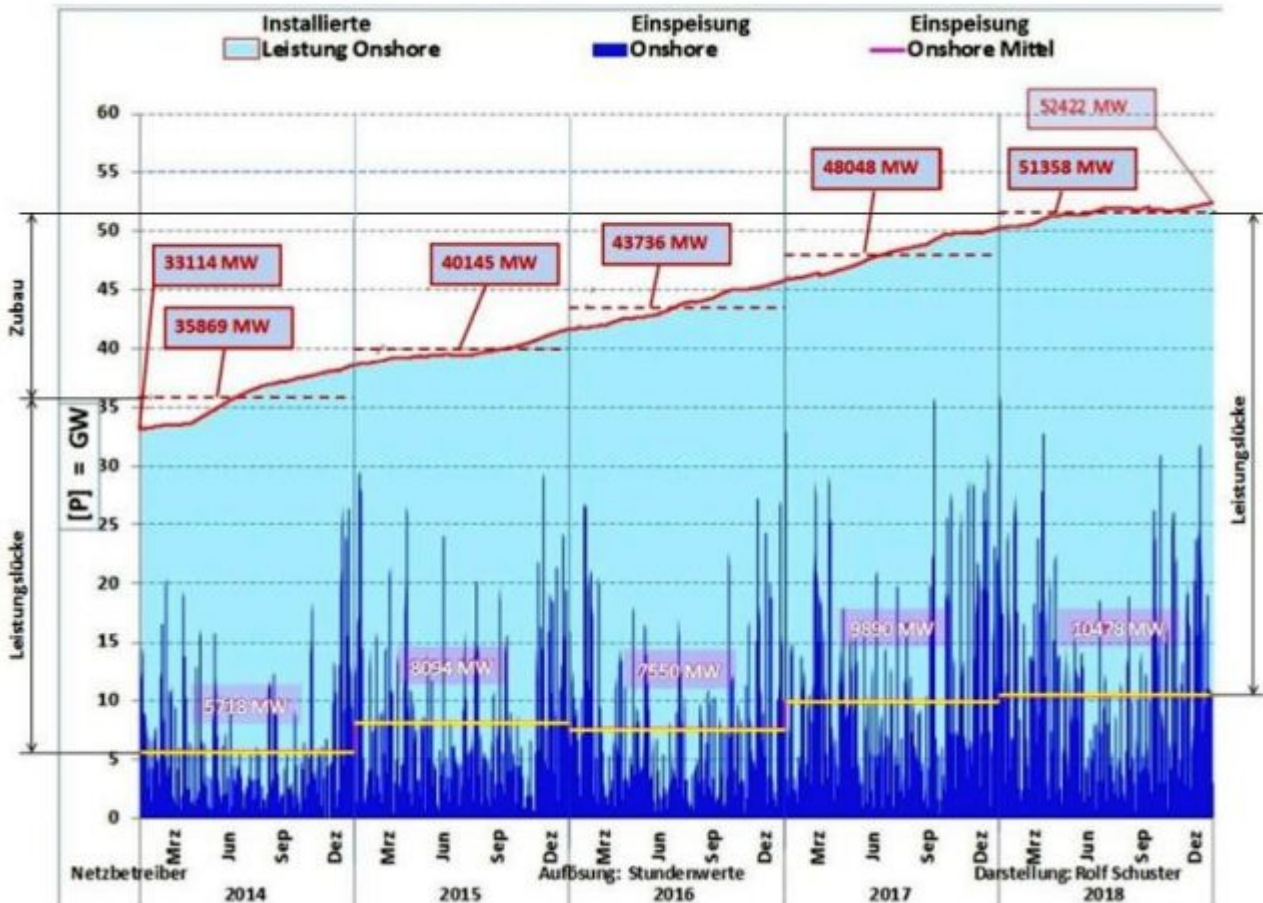
Rolf_Schuster_ Nennleistung vs Kapazität
