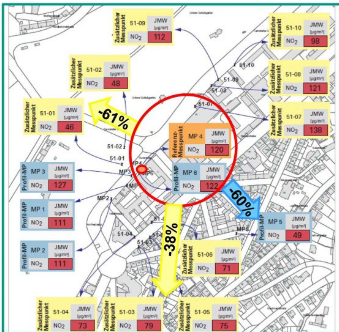
Bild 3. Schon in vergleichsweise geringer Entfernung von „Am Neckartor“ (kleiner roter Kreis) zeigen andere Messstationen NO2-Jahresmittelwerte an, die um 38 oder sogar 60 % niedriger liegen (Grafik: IFKM/ KIT)
