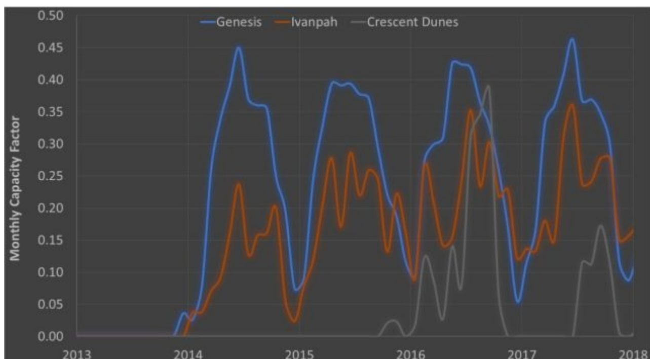
Solarkraftwerke-Kapazitätsfaktoren- Quelle NREL
