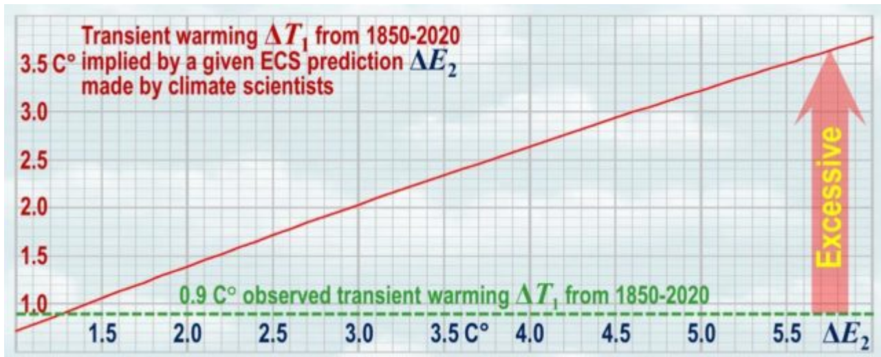
Abbildung 12: Alle derzeitigen Prognosen der Enderwärmung (ECS) von 2^\circ\text{C} oder mehr aufgrund einer \text{CO}_2 -Verdoppelung im Zeitraum 1850 bis 2020 liegen weit über den gemessenen 0,9^\circ\text{C} .
