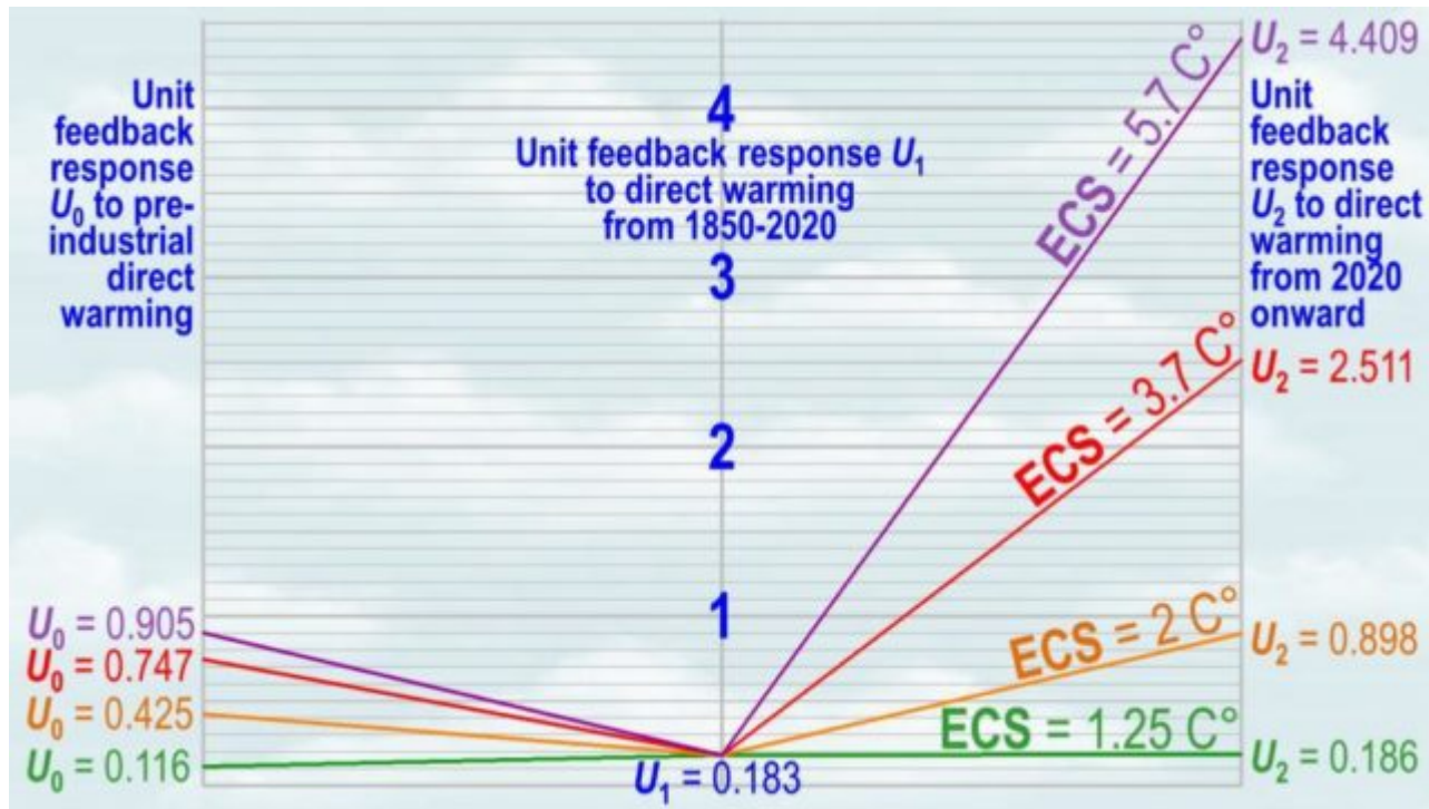
Abbildung 11: Rückkopplungs-Reaktionen der Einheit U_0 \leq U_1 \leq U_2 (solche pro 1^\circ\text{C} direkter Treibhauserwärmung) sollten mit der Erwärmung zunehmen. Sie tun genau das unter der Annahme einer Enderwärmung von 1,25^\circ\text{C} durch verdoppeltes \text{CO}_2 (equilibrium climate sensitivity, oder ECS: die grüne Linie). Basierend auf der vorhergesagten \text{ECS} \geq 2^\circ\text{C} in aktuellen Klimamodellen geht die Reihe jedoch unweigerlich nach unten statt nach oben.
