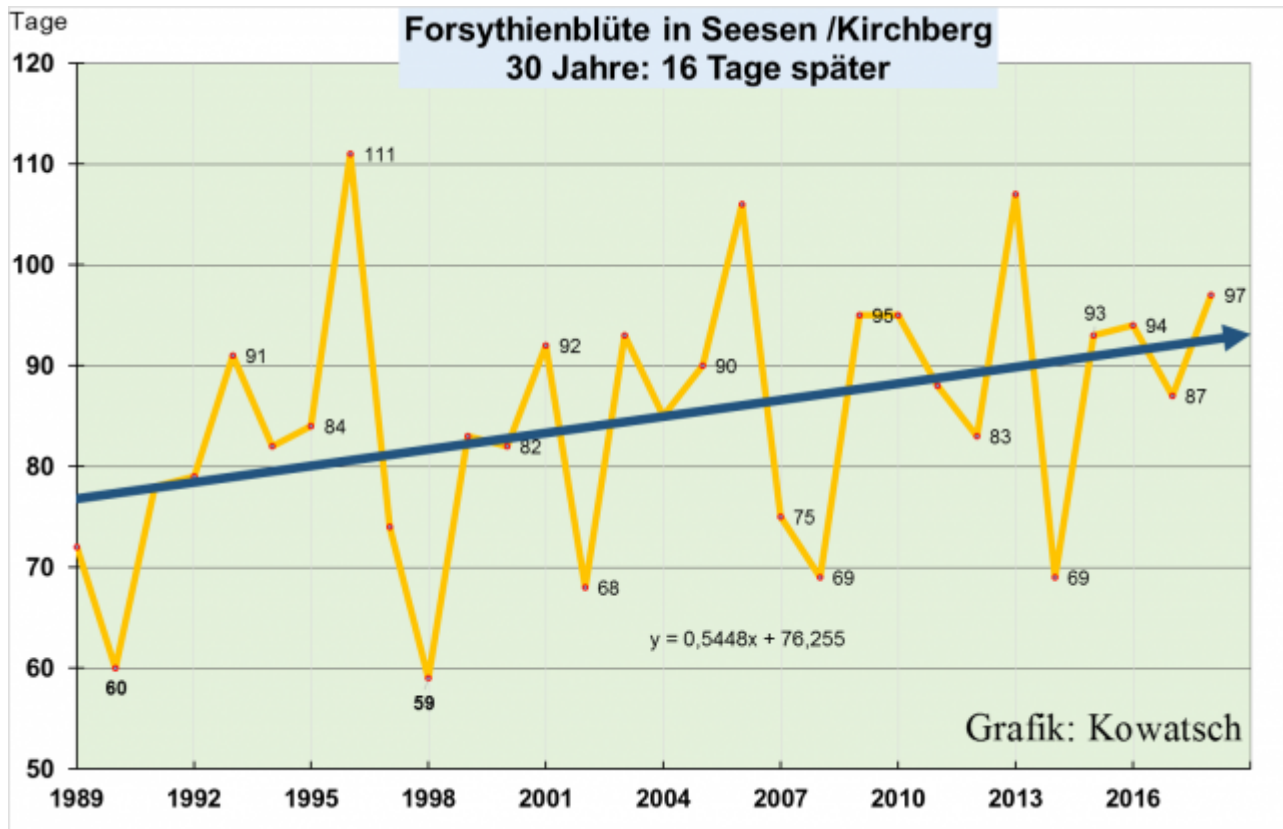
Grafik 1: Ähnlich wie der Frosythienstrauch in Hamburg verspätet sich seit 30 Jahren auch der Forsythienstrauch in Seesen. Steigende Trendlinie bedeutet Verspätung. In der Grafik sind als Blühtermin die Tage ab Neujahr angegeben.
