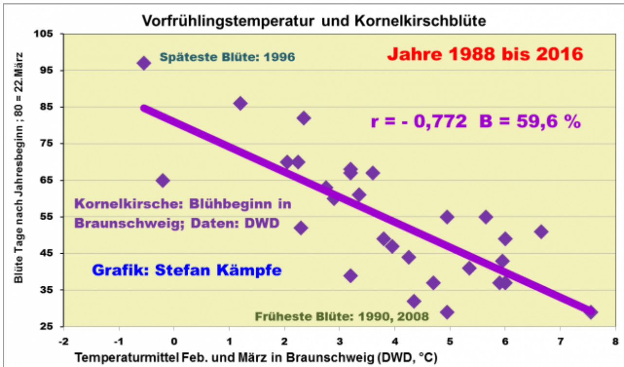
Grafik 5: Ein kälterer Vorfrühling zieht tendenziell eine längere Dauer bis zum Beginn der Kornelkirschblüte nach sich (negative Korrelation). Man beachte aber, dass außer der Lufttemperatur auch die Sonnenscheindauer, die Bodentemperatur, die Bodenfeuchte und die gestiegene CO 2 -Konzentration der Atmosphäre einen wesentlichen Einfluss auf den Zeitpunkt des Erblühens haben!
