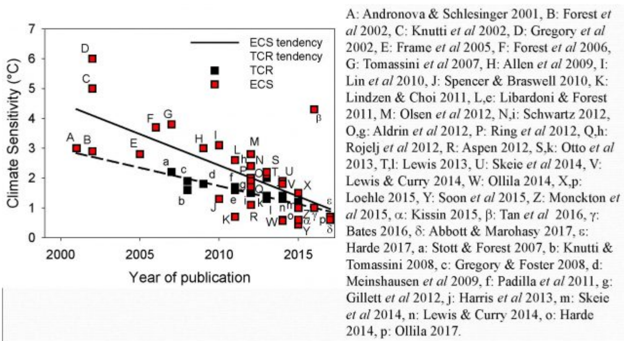
Bild 2: Klimasensitivität (ECS und TCR) in der begutachteten Fachliteratur über die Jahre ( Bildquelle: F. Gervais, zuerst veröffentlicht hier , danach von ihm ergänzt auf der EIKE-Klimakonferenz in Düsseldorf 2017 auf der Basis jüngster Fachpublikationen hier ). Es ist eine eindeutige Tendenz zu unbedenklich kleinen Werten der Klimasensitivität ( = globale Erwärmung bei hypothetischer Verdoppelung des atmosphärischen CO 2 -Gehalts ) zu erkennen.
