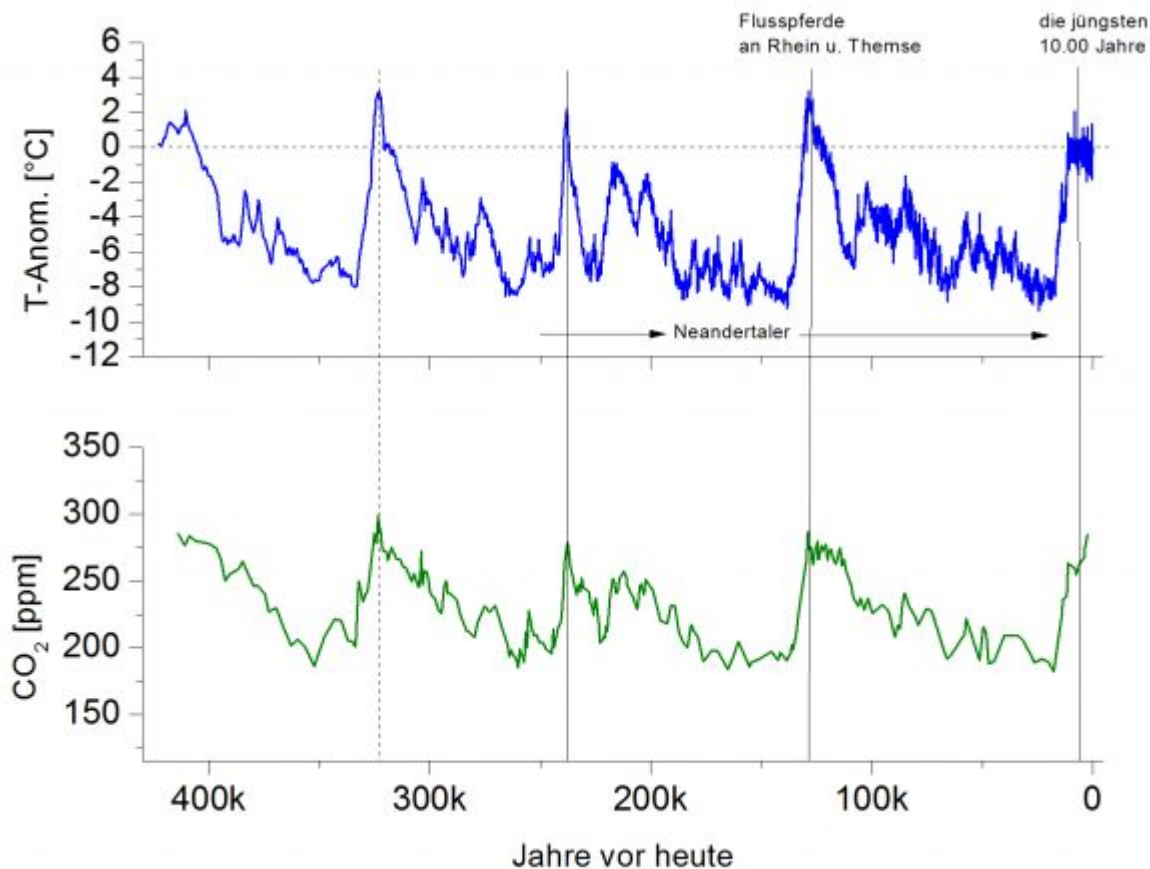
Abb. 2: Vostok-Eisbohrkernkurve, nach [5] Petit et al. 1999, Nature 399, Fig. 3. Relevant ist hier der kurze Verlauf der letzten 10.000 Jahre in der Gesamtkurve (blau oben rechts): Man erkennt im Holozän, insbesondere bei besserer Zeitauflösung als in dieser Abbildung, mehrere Temperaturmaxima höher als heute.
