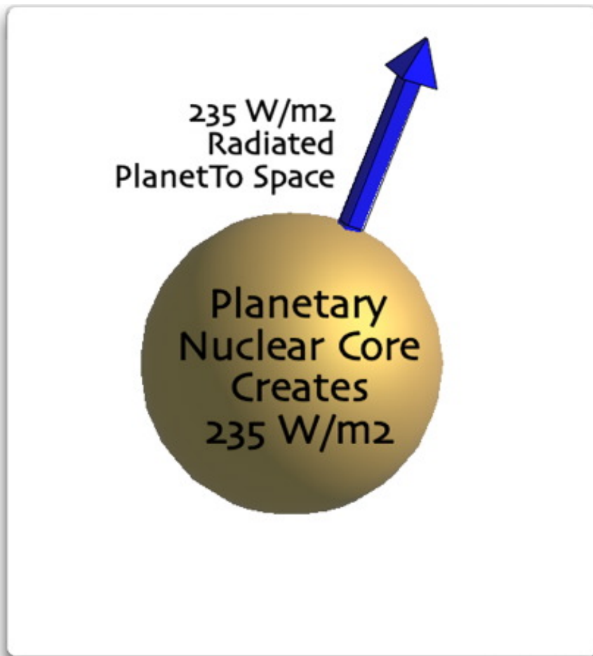
Abbildung 1: Planet im freien Weltraum, erwärmt aus seinem Inneren. Die Zeichnung zeigt die Lage im Gleichgewicht.
