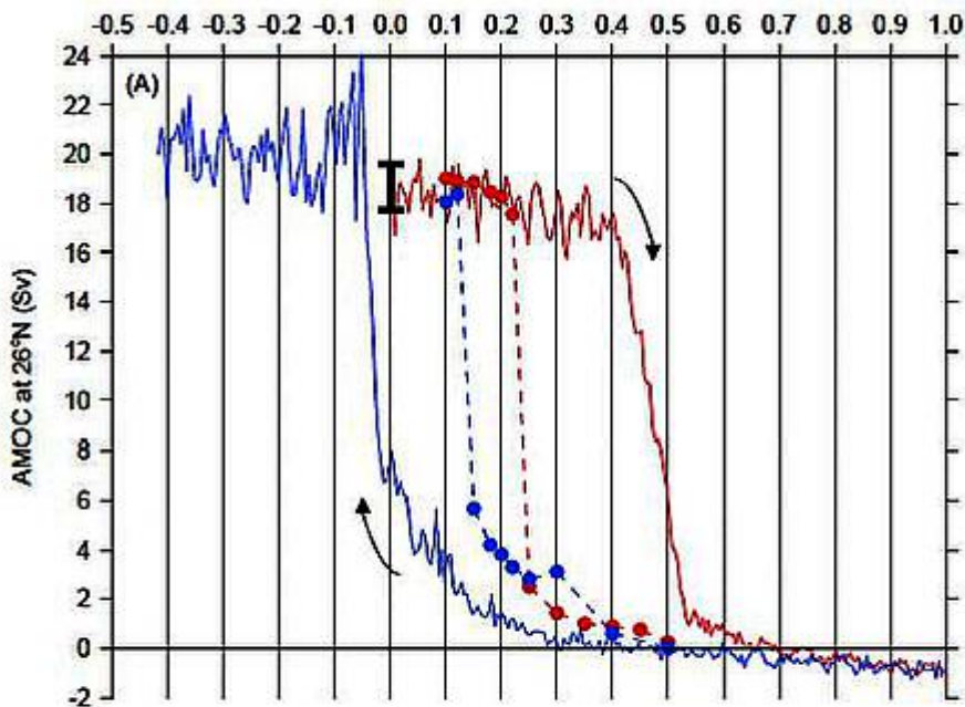
Bild 3: Die Stärke der AMOC in Abhängigkeit des natürlichen Zu/Abflusses an Süßwasser im Südatlantik. Es gibt zwei Zustände (Bistabilität) mit Hysterese, das „Ausschalten“ ist in rot gezeichnet, das „Einschalten“ in blau. Quelle: Bild 2 der o.g. Arbeit.
