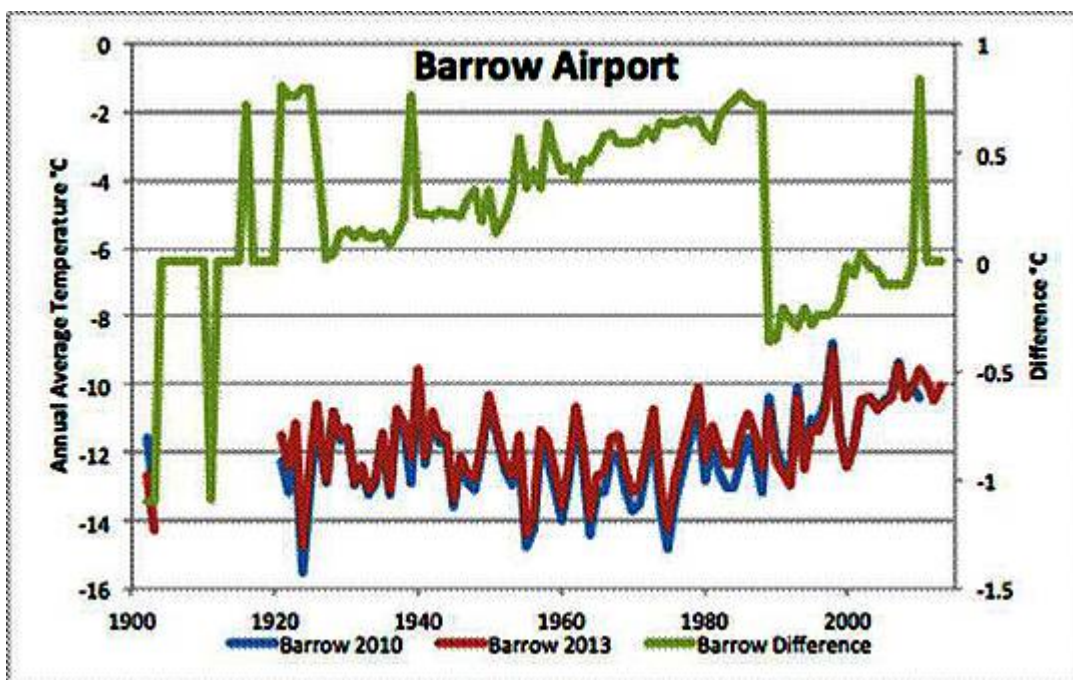
Abbildung 2: Plot der jährlichen Temperatur in Barrow, Alaska,
