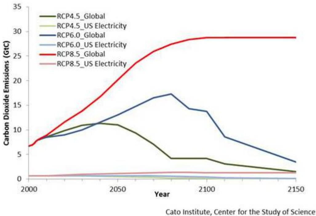
Abbildung 1: Verlauf von CO 2 -Emissionen definiert nach oder abgeleitet aus dem Original-Satz von RCPs, und zwar für die globalen Gesamt-CO 2 -Emissionen ebenso wie für die CO 2 -Emissionen, die der US-Stromerzeugung geschuldet sind.
