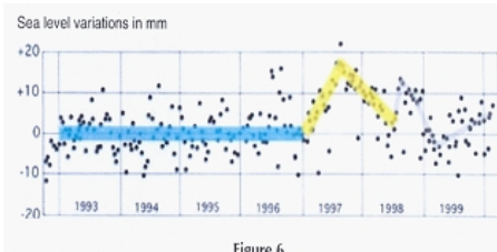
Abbildung 6 Änderungen des Meeresspiegels aus Abbildung 5 mit Berücksichtigung der ENSO-Spitze
