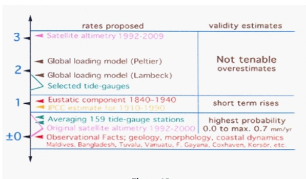
Abbildung 12 Evaluierung der Zuverlässigkeit für verschiedene behauptete Meeresspiegelraten
