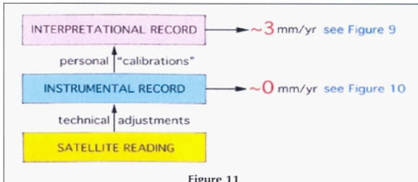
Abbildung 11 Satellitenmessungen und die zwei Arten von angebrachten Korrekturen
