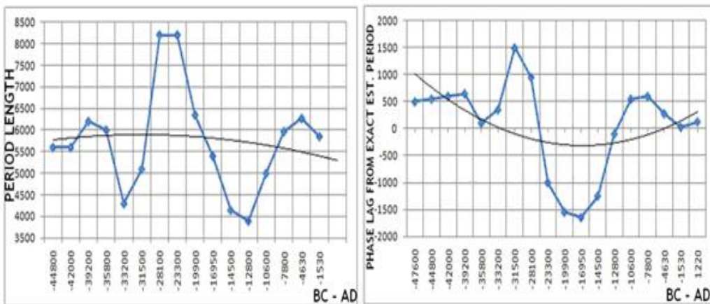
Abbildung 202: Periodenlänge (links) und Phasenverschiebung (rechts) des 5.800 Jahres-Zyklus, der Einfluss auf den 200- und den 2.300-Zyklus hat, Quelle:
