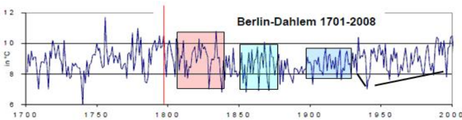
Abbildung 188: Temperaturangreihe von Berlin-Dahlem von 1701 – 2008 mit den gleichen Merkmalen.
