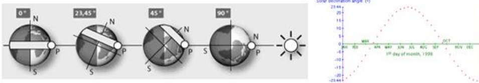
Abbildung 201 (Quelle: www.Biosphaere.info ) zeigt die Lage der subsolaren Zone (Sonne steht senkrecht am Firmament) zur Obligität und die Abbildung rechts die ihre tatsächliche Wanderung über das Jahr, Quelle: ( http://joseph-bartlo.net/supp/sungeo.htm ).
