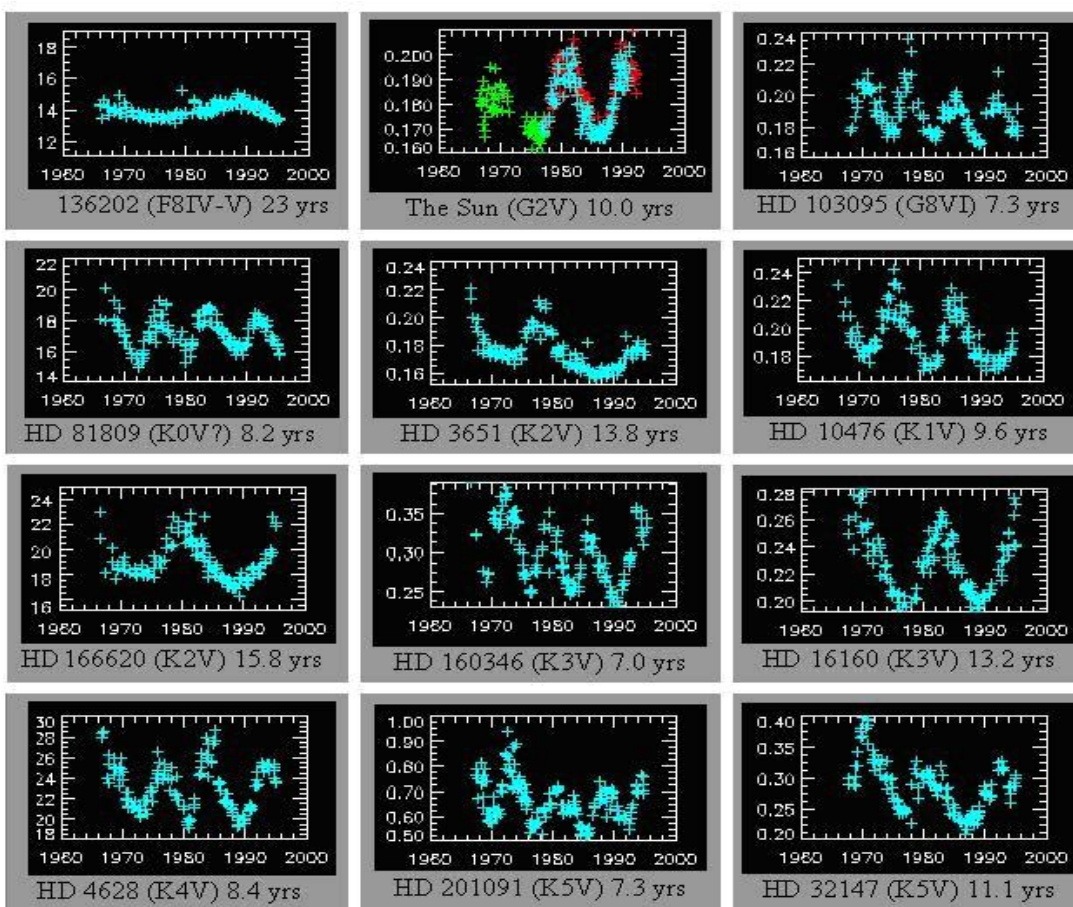
Abbildung 214, Quelle: ( http://solar.physics.montana.edu/reu/2004/awilmot/introduction.html ), zeigt am Beispiel von 11 Sternen, dass diese ähnliche Muster in ihren Aktivitätsschwankungen wie die Sonne (oben Mitte) aufweisen, was auf magnetische Aktivitätszyklen zurückzuführen ist und die
