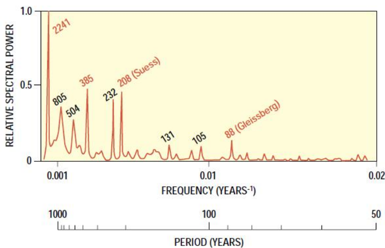
Abbildung 199, Quelle: United States Geological Survey, "The Sun and Climate", August 2000, zeigt das Energiespektrum der 14C-Daten. Deutlich sind Maxima zu erkennen, die Sonnenzyklen zuzuordnen sind.
