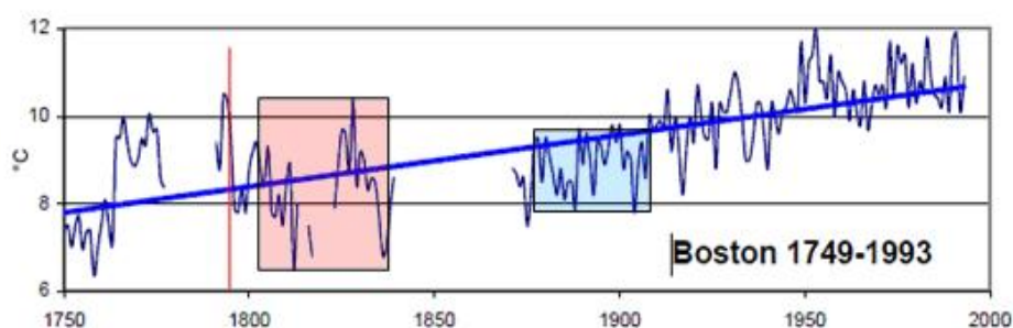
Abbildung 192: Nicht nur in Europa, sondern auch in Amerika ergibt sich das gleiche Muster des Temperaturganges nach einem Hauptsonnenzyklus, wenn auch hier sozusagen der mittlere Teil fehlt, weil keine Messungen vorhanden sind.
