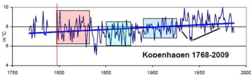
Abbildung 184, Quelle: Prof. Ewert, EIKE, zeigt den Temperaturgang von Kopenhagen im Zeitraum von 1768 - 2009. Die rote Linie gibt den Zeitpunkt des Maximums im Hauptsonnenzyklus an. Bis zu einem Zeitraum von 20 - 30 Jahren nach dem Hauptsonnenzyklus schwanken die Temperaturen noch stark zwischen warm und kalt (rote Fläche). Bis zum Erreichen seines Minimums, sind immer noch relativ hohe Temperaturschwankungen zu verzeichnen, jedoch auf insgesamt niedrigerem Niveau (grüne Fläche). Unmittelbar vor und nach dessen Minimum ist das Klimasystem sozusagen in seinem eingeschwungenen, kalten Zustand und die Schwankungen sind am geringsten (blaue Fläche). Vor einem erneuten Temperaturanstieg (steigender Sonnenzyklus), fallen die Temperaturen auf ein Minimum und steigen dann kontinuierlich an (schwarze Linien).
