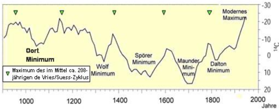
Abbildung 183 zeigt die Kälteperioden der letzten 1.100 Jahre (ergänzt nach Quelle: United States Geological Survey). Die Maxima der Warmperioden korrelieren jeweils mit dem Maximum des de Vries/Suess-Zyklus. Nach jedem Maximum fallen die Temperaturen deutlich.
