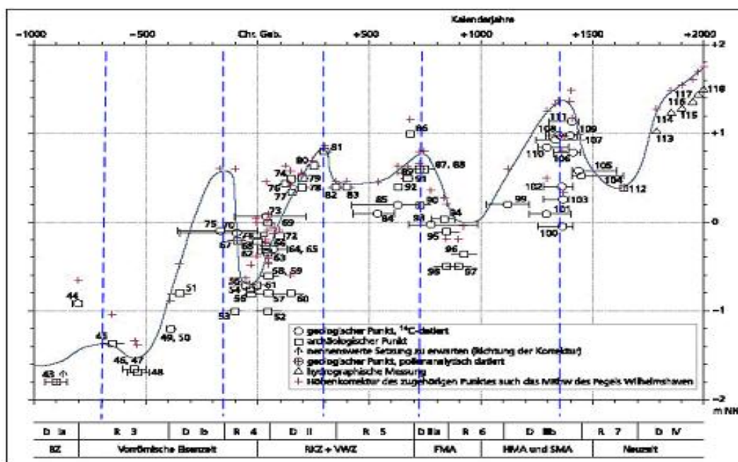
Abbildung 200, Quelle: K.E. Behre, "Probleme der Küstenforschung", Band 28, Isensee-Verlag, 2003,
