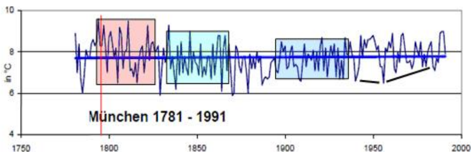
Abbildung 187: Ebenfalls das gleiche Bild bei der Temperaturgangreihe München im Zeitraum von 1781 - 1991.
