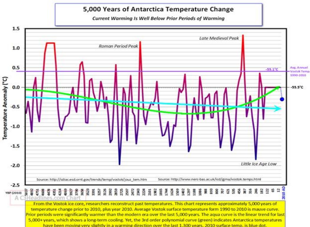
Abbildung 198 zeigt den Temperaturgang in der Antarktis der letzten 5.000 Jahre
