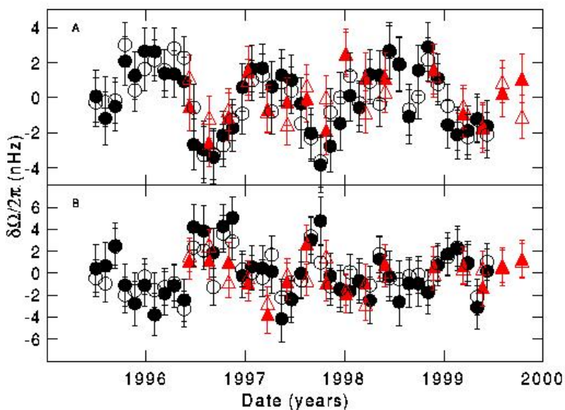
Abbildung 213, Quelle: ( http://soi.stanford.edu/press/GONG_MDI_03-00/pressbase.gif ) zeigt die Oszillation im Sonneninneren ( 0,72 Sonnenradius oben und 0,63 Sonnenradius unten). Deutlich die die 16-Monatsschwingung zu sehen und dies in Gebieten, über die Tachocline hinaus. Das darin enthaltene Gas rotiert mal schneller und mal langsamer. Rot sind nach MDI (Michelson Doppler Imager, SOHO) und schwarz nach GONG-Daten (Global Oscillation Network Group). “Entdeckt wurden die von niemand vorausgesagten Strömungen in vierjährigen Meßreihen des MDI-Instruments auf dem Satelliten SOHO und des GONG-Netzes von Sonnenteleskopen rund um die Erde.” ( http://www.astro.uni-bonn.de/~dfischer/news/SuW-L-1-10.html )
