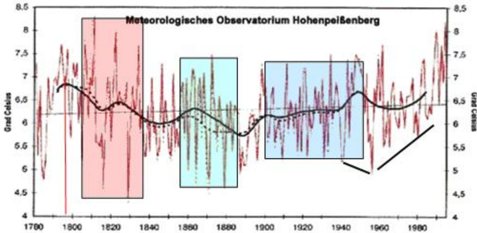
Abbildung 185, Quelle: ( http://www.lanuv.nrw.de/luft/wirkungen/klima_grundlagen.htm ) zeigt den Temperaturgang des Hohenpeißenberg von 1781-1995 nach Fricke 1997. Die rote Linie kennzeichnet wieder das Maximum des Hauptsonnenzyklus. Auch hier sind bis 30 Jahre nach dem Hauptsonnenzyklus starke Jahresschwankungen der Temperatur zu sehen (rote Fläche), die dann geringer werden (grüne Fläche) und nach dem Minimum im Hauptsonnenzyklus die geringsten Werte einnehmen (blaue Fläche).
