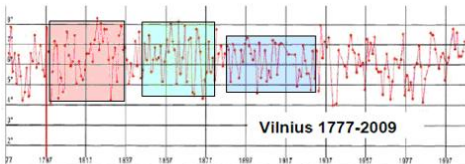
Abbildung 191: In Vilnius ein ähnliches Bild.
