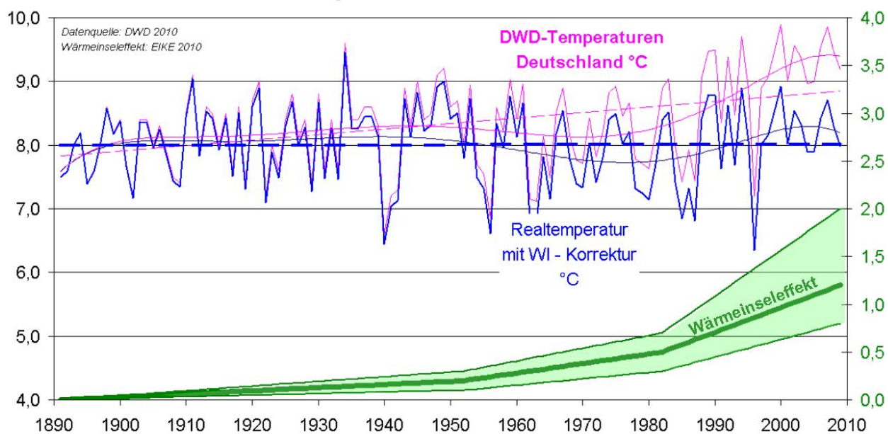
Die Deutschlandtemperaturen des DWD 1891 -2009
