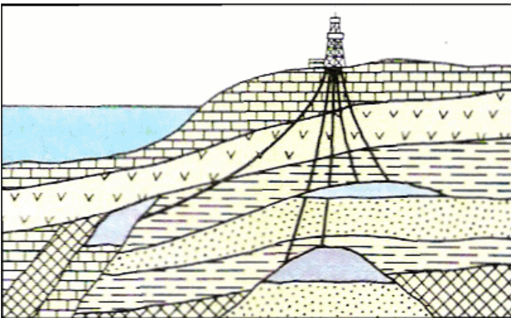
Abb. 3: Beispiel für gerichtetes Bohren („Nestbohren“) von einem Punkt aus (nach „Bergencyklopädie“ V3, S. 137 – Kozlowski et. al (Red.), Moskau 1987)
