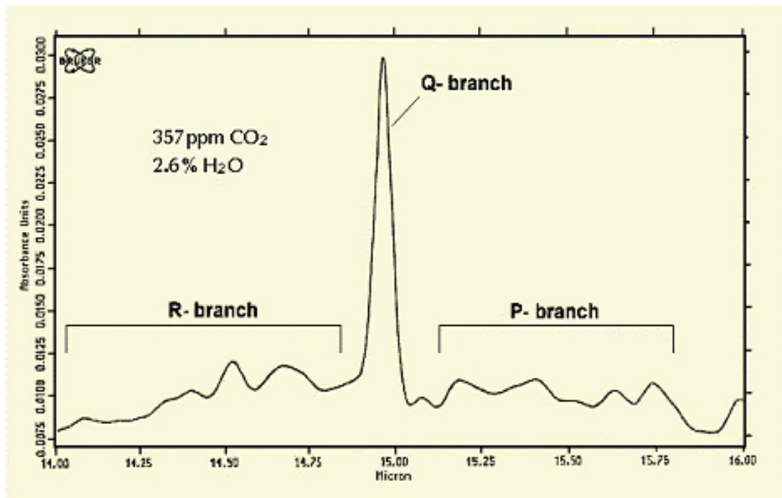
(Bild 4: Unbearbeitetes Spektrum der 15 \mu m-Bande ( \nu_2 -Bande))
