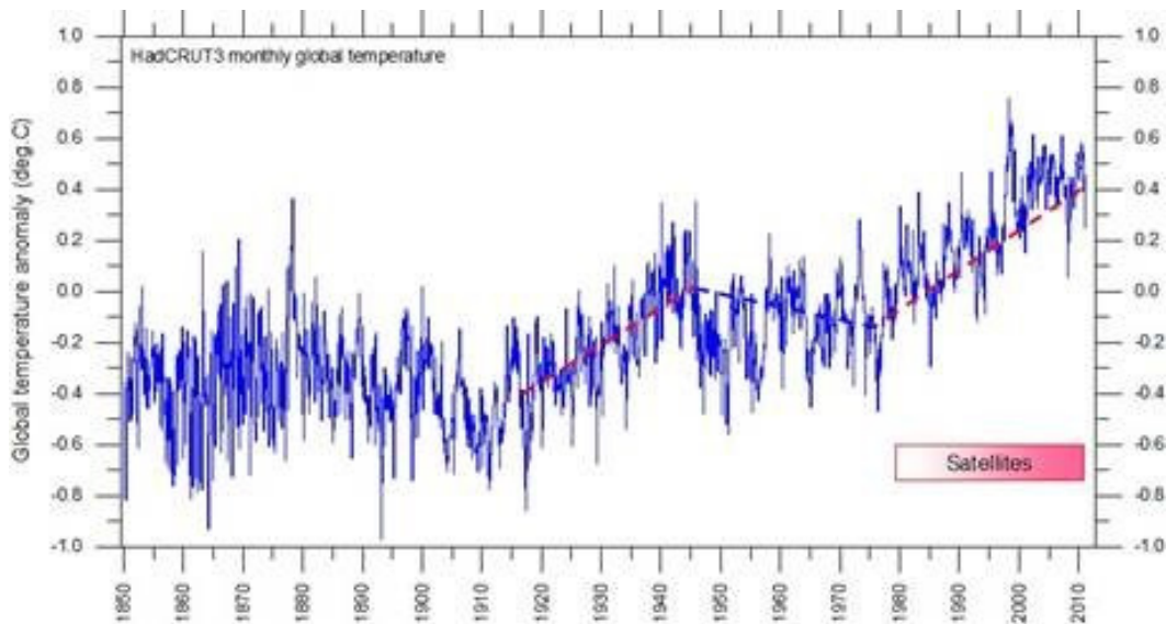
Abbildung 4: Globale Temperatur im vergangenen Jahrhundert.
