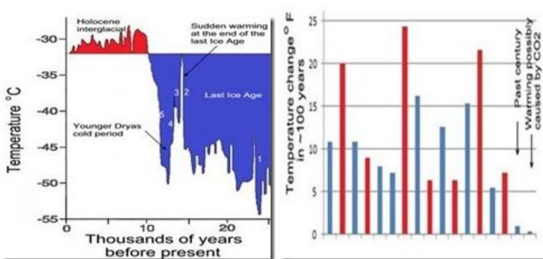
Abbildung 5: A: Temperaturänderungen im GISP2-Eisbohrkern vom Ende der letzten Eiszeit während des Holozäns. (Easterbrook 2011, modifiziert aus Cuffy und Clow 1997). B: Raten von Temperaturänderungen (Easterbrook 2011).
